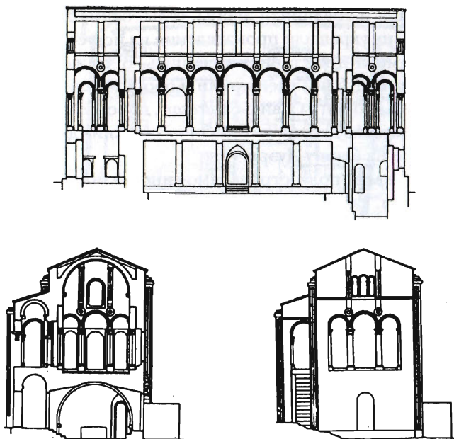
Дворец Наранко: проекция и поперечный разрез
