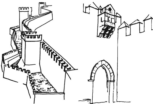
Стена и барбакан, навесные бойницы
