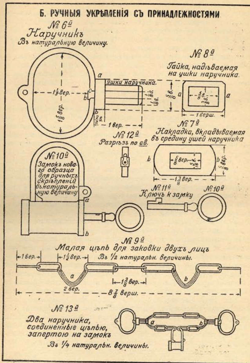
Рис. 4. Ручные скрепы
