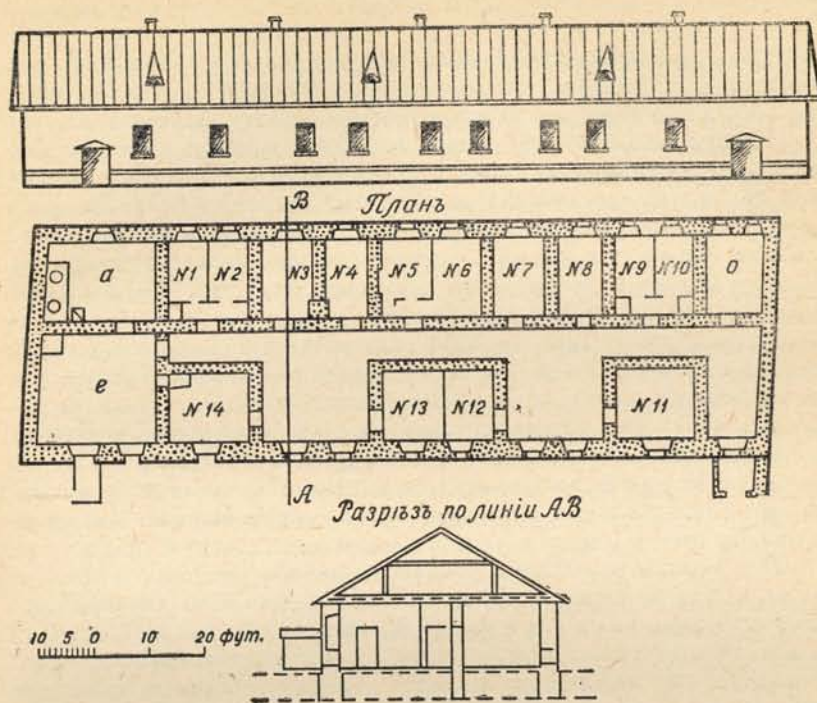
Рис. 13. Шлиссельбургская крепость в 1881 г. План старой тюрьмы для политических заключенных. Из дела ЦГИА в Москве.
