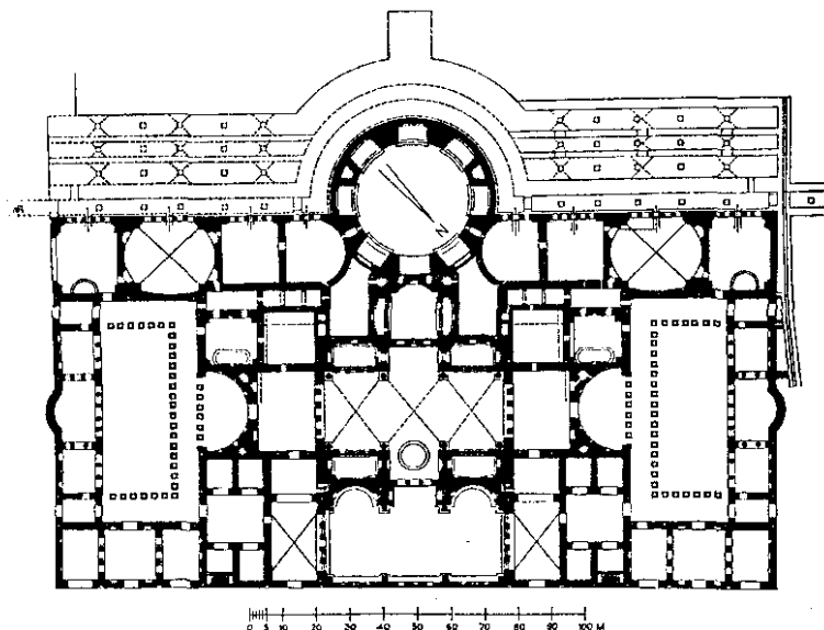
Рис. 49. Термы Каракаллы. Рим (горизонтальная проекция)
