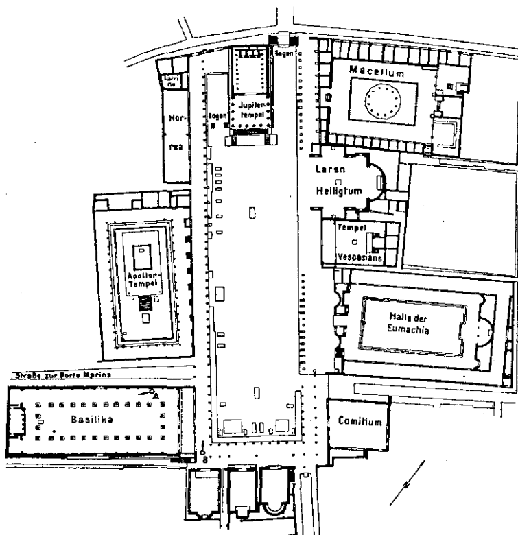
Рис. 43. Форум Помпей, горизонтальная проекция
