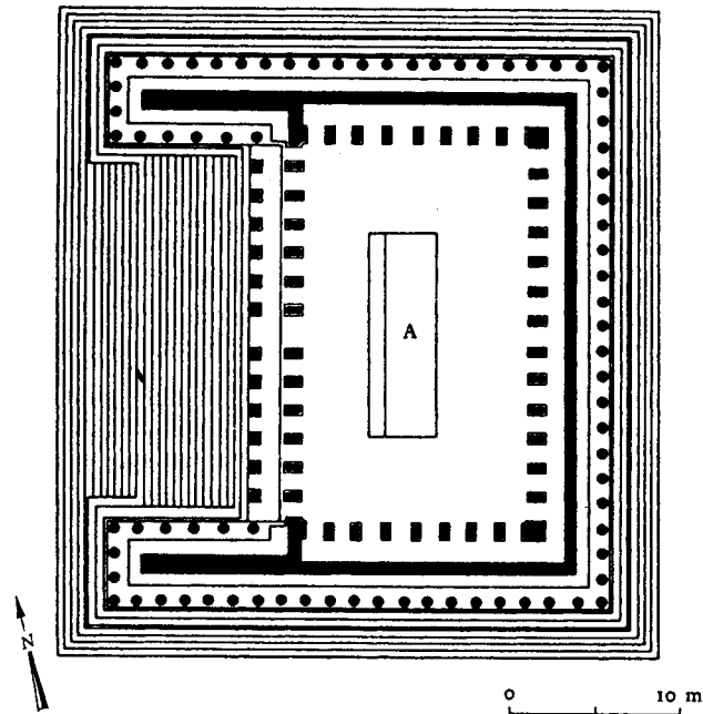
19. Большой пергамский жертвенник
