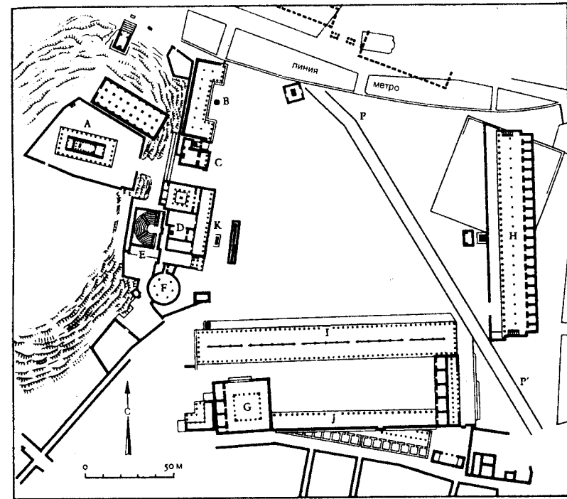
11. Афинская агора в конце эллинистической эпохи
