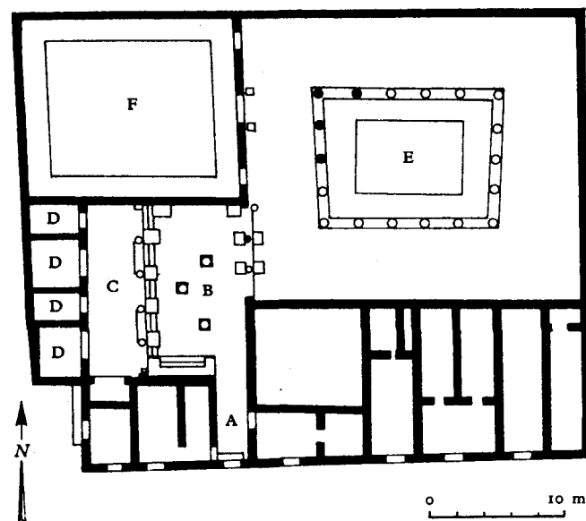
8. Делос: дом беритских посейдониастов
