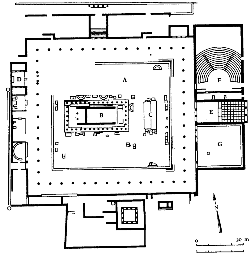
15. Мессена: план агоры
