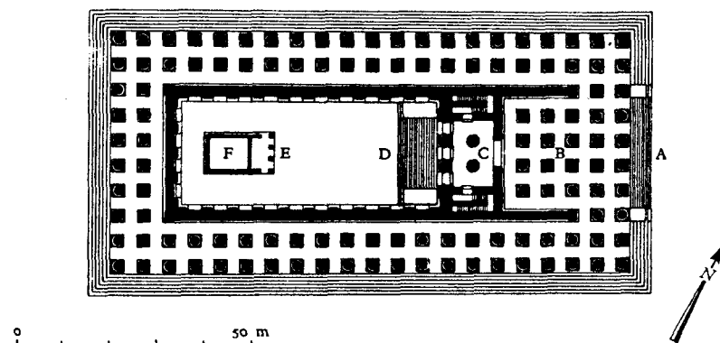
17. Храм Аполлона в Дидимах
