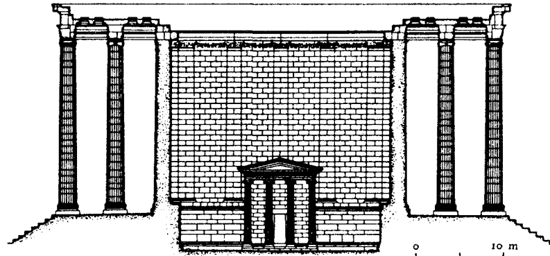
18. Храм Аполлона в Дидимах: поперечный разрез
