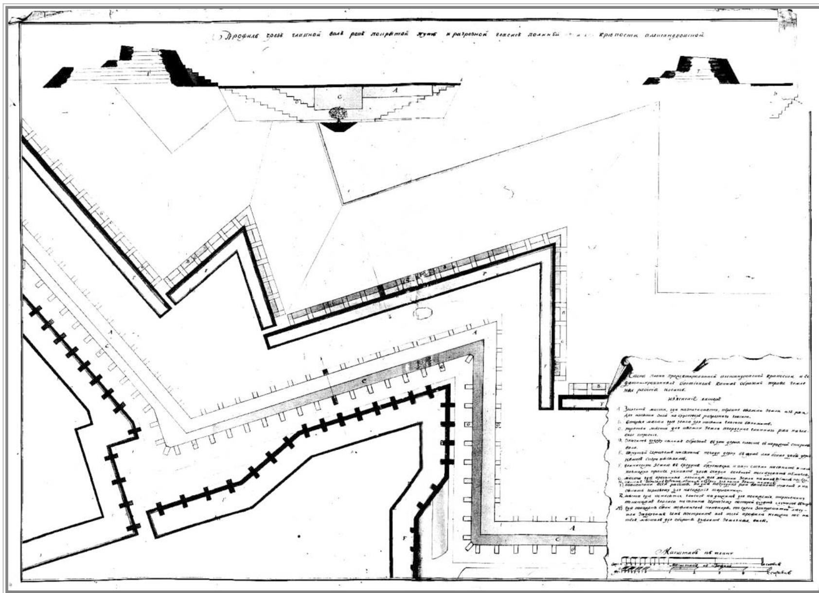
Часть плана проектируемой крепости Александровской. 1770–1771 гг. ЗОУНБ (коллекция В.Г. Фоменко)
