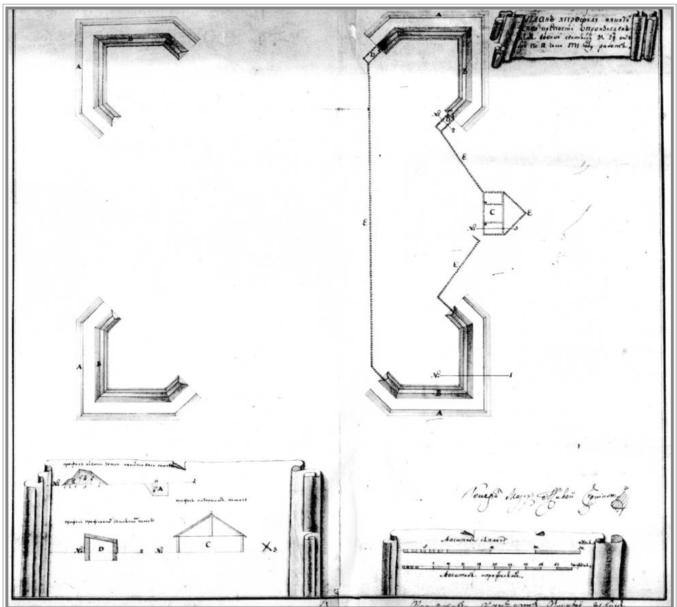
План крепости Никитинской (1-й) с показанием произведенных в ней работ с 24 сентября по 18 октября 1771 г. ЗОУНБ (коллекция В.Г. Фоменко)
