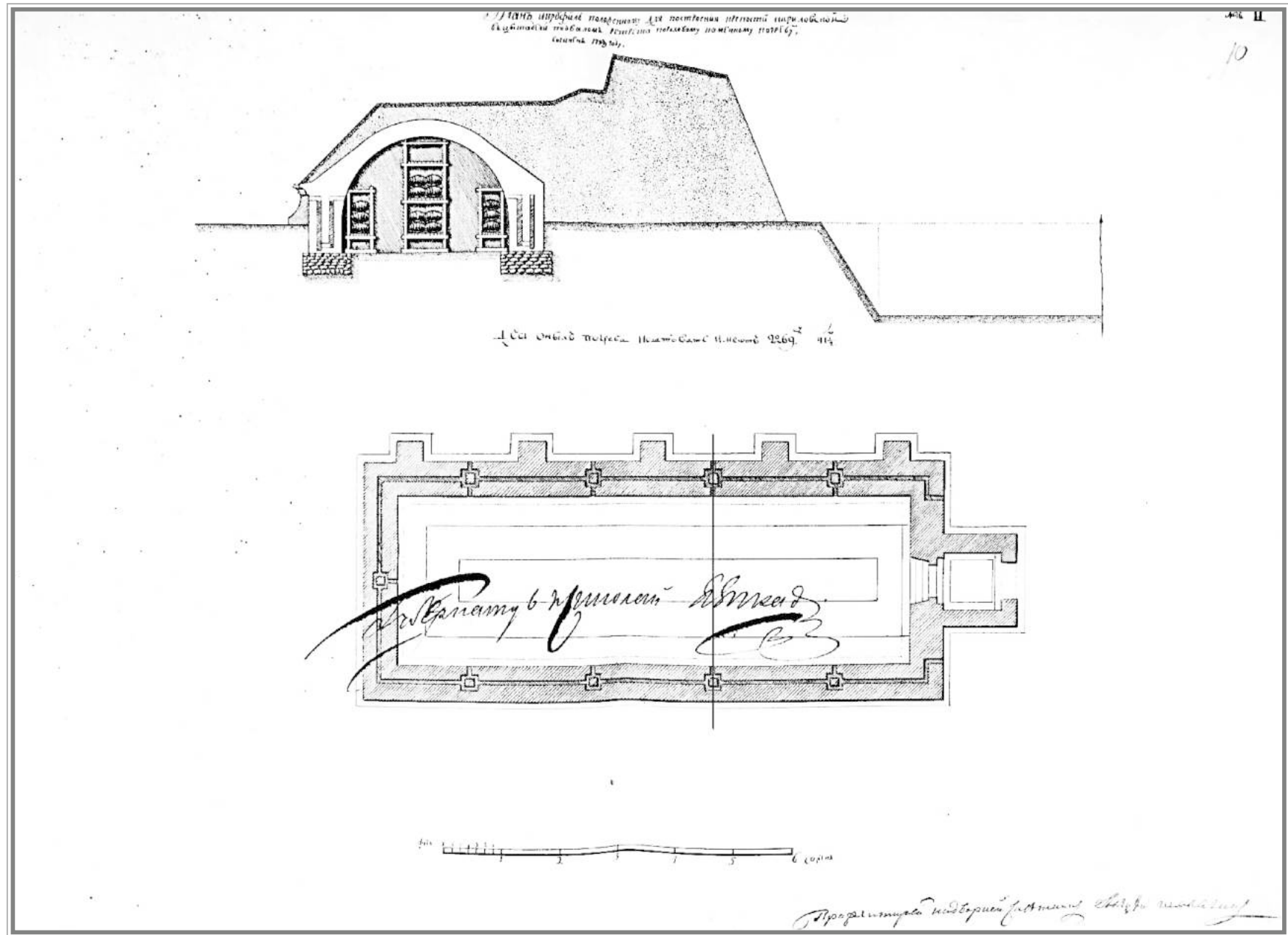
План проекта порохового погреба в цитадели крепости Кирилловской. 1783 г. ГАРК, ф. 535, оп. 1, д. 3152
