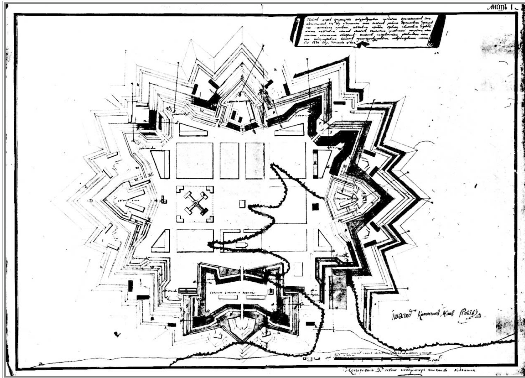
План крепости Александровской с показанием выполненных в ней работ. 4 декабря 1774 г. ЗОУНБ (коллекция В.Г. Фоменко)
