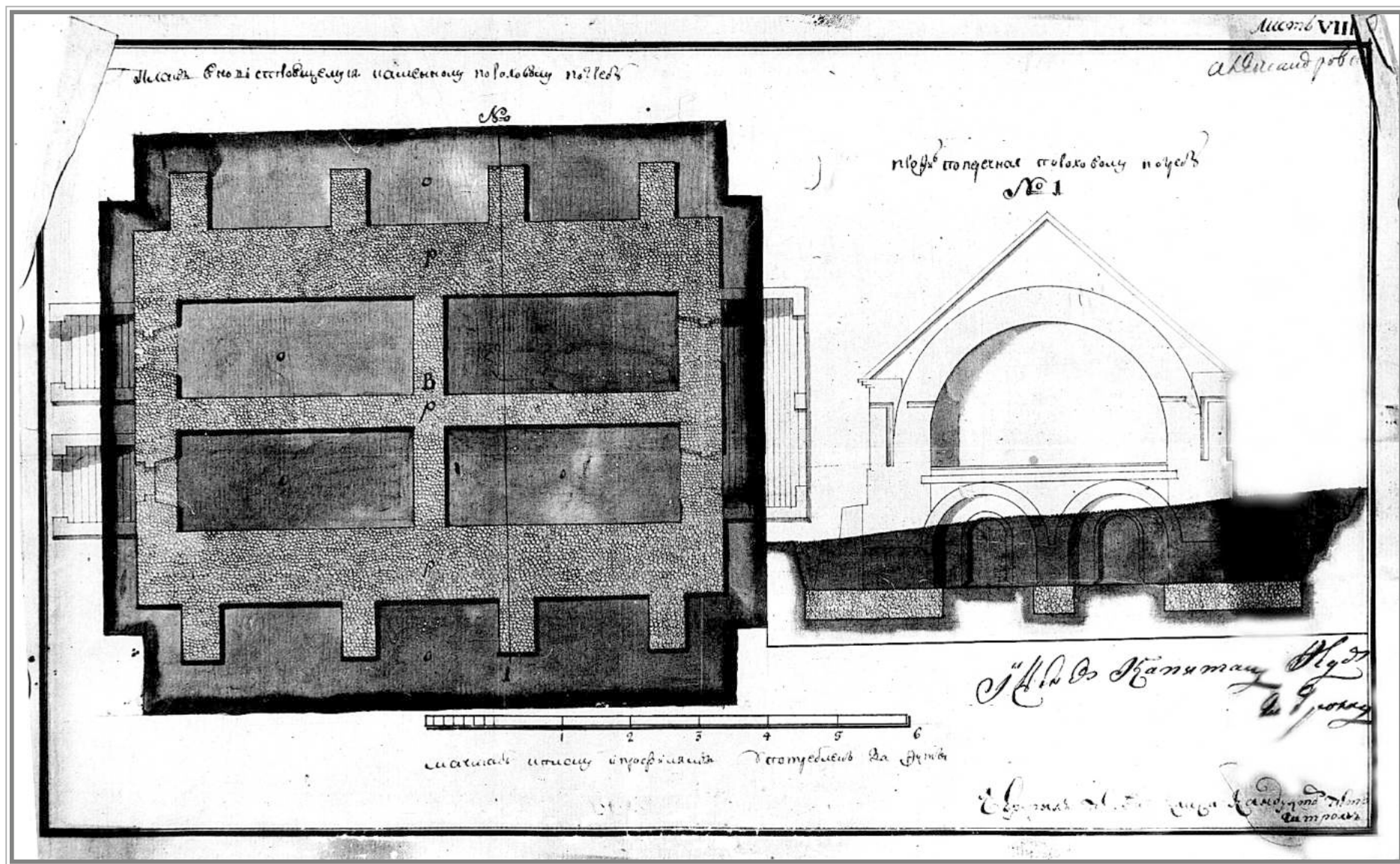
План строящегося порохового погреба в крепости Александровской. 1770-е гг. ЗОУНБ (коллекция В.Г. Фоменко)
