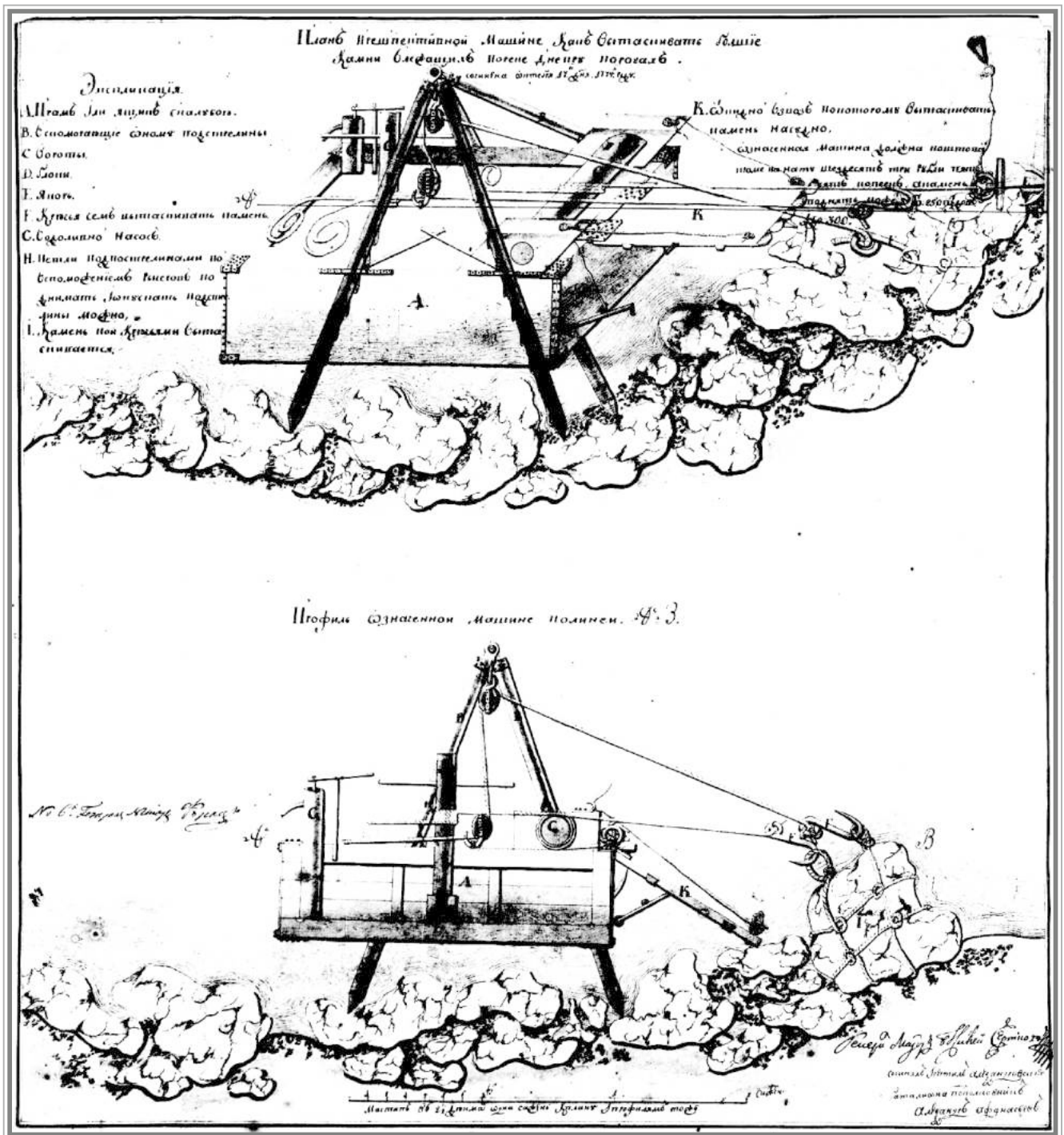
Проект машины для вытаскивания камней на Днепровских порогах, сделанный командиром Александровского пограничного батальона подполковником А. Афанасьевым. РГВИА, ф. 349, оп. 12, д. 5060
