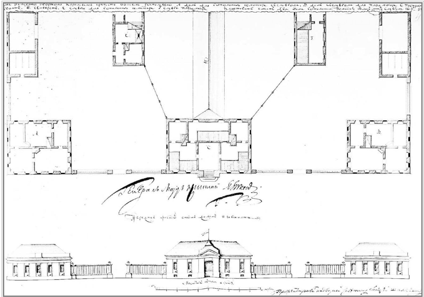
План проекта квартала, в котором расположены дома для батальонного командира и плац-майора крепости Кирилловской. 1783 г. ГАРК, ф. 535, оп. 1, д. 3152
