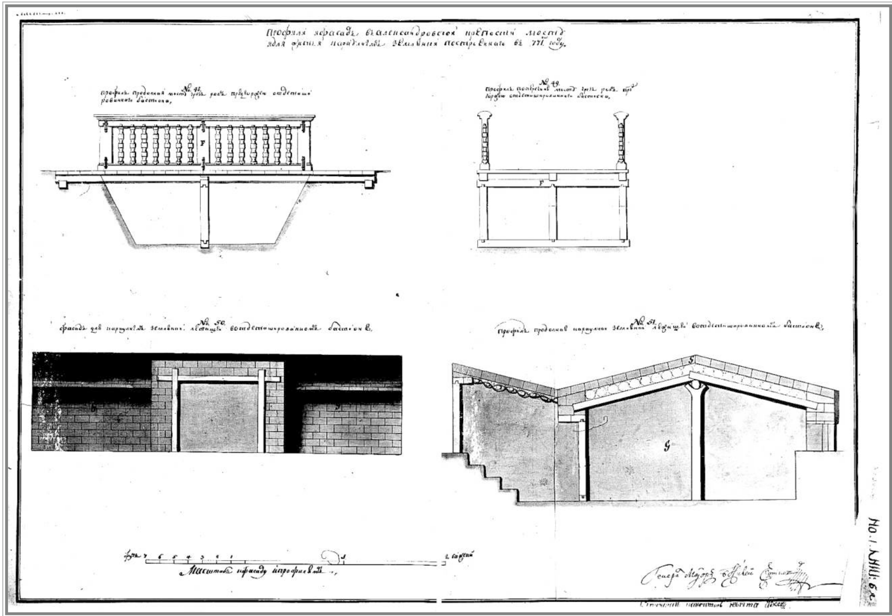
Профили и фасады караульной землянки и моста через ров в крепости Александровской. 1771 г. ЗОУНБ (коллекция В.Г. Фоменко)
