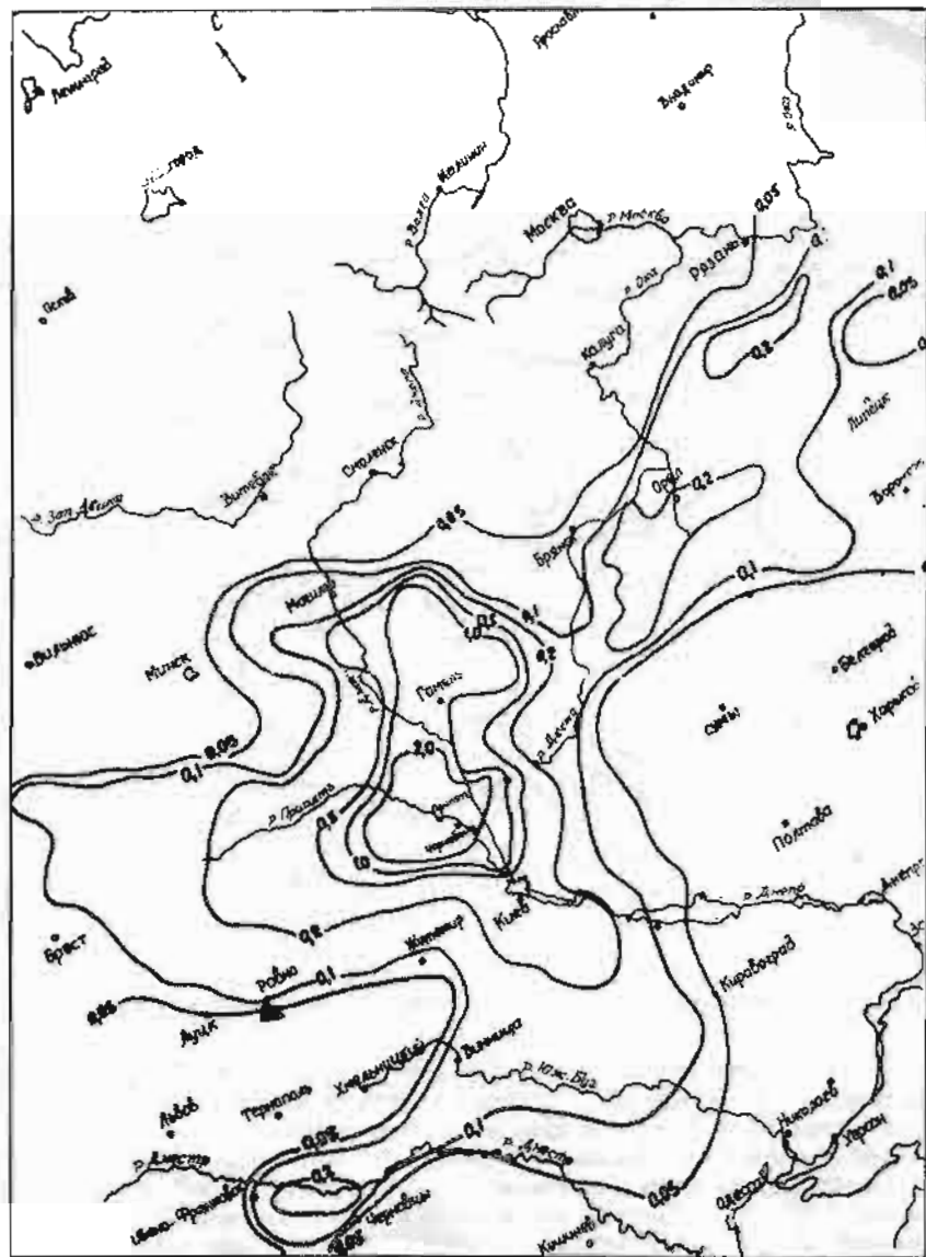
рис. 8.6 Результаты гамма-съемки Европейской части СССР в первые дни после аварии (МР/4)
