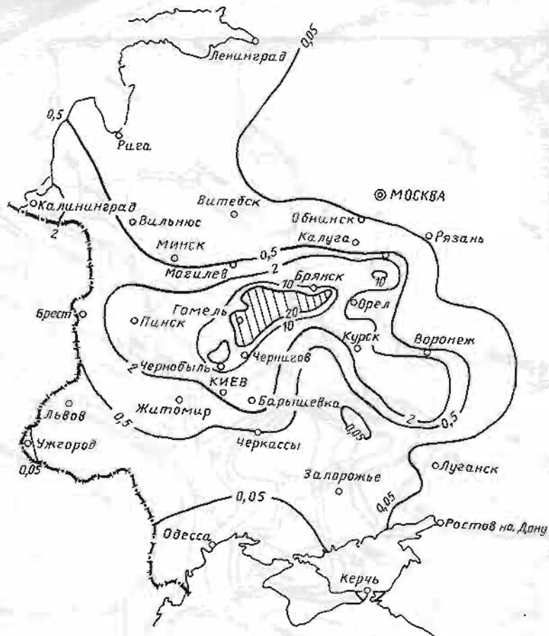
рис. 8.5 Плотность выпадения иода-131 на почву, приведенная на 15 мая 1986г. (Ки/км 2 )
