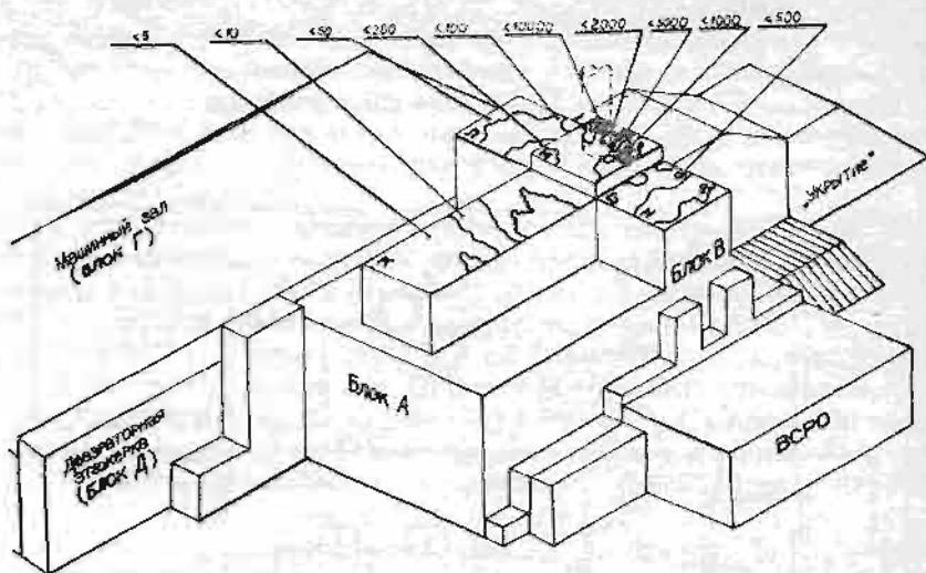
рис. 8.2 Уровни радиации (P/ч) на крыше II очереди ЧАЭС (лето 1986г.)
