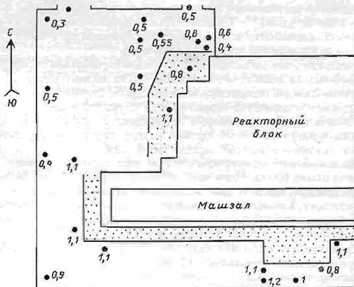
рис. 8.3 Уровни радиации (P/ч) на промплощадке ЧАЭС к моменту завершения строительства объекта "Укрытие"
