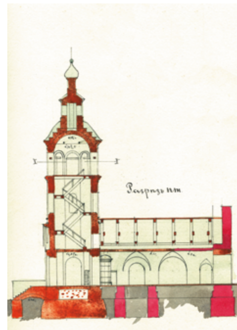
Чертёж в разрезе. Из фондов Чердынского краеведческого музея им. А.С. Пушкина
