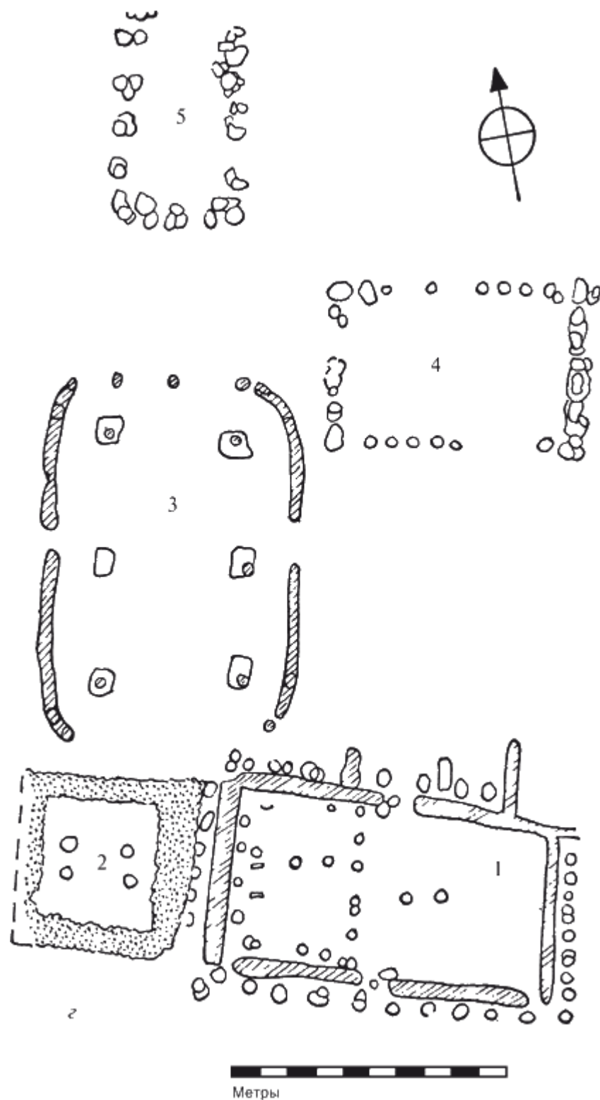
Рис. 9. a – план королевского жилища в Иверинге (по Хоуп-Тейлору); б – план здания в виде лодки в Чеддере; в – второй по величине дом в XII столетии в Чеддере; г – примерный план комплекса зданий в Портчестере.
