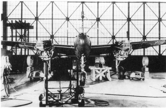
«Лайтнинг» во время статических испытаний прочности в ЦАГИ. Двигатели заменены балластом
