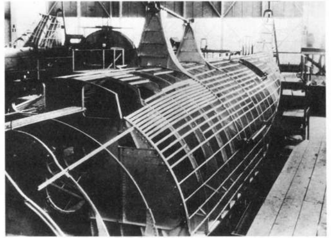
Сборка американских летающих лодок в Таганроге, декабрь 1938 года
