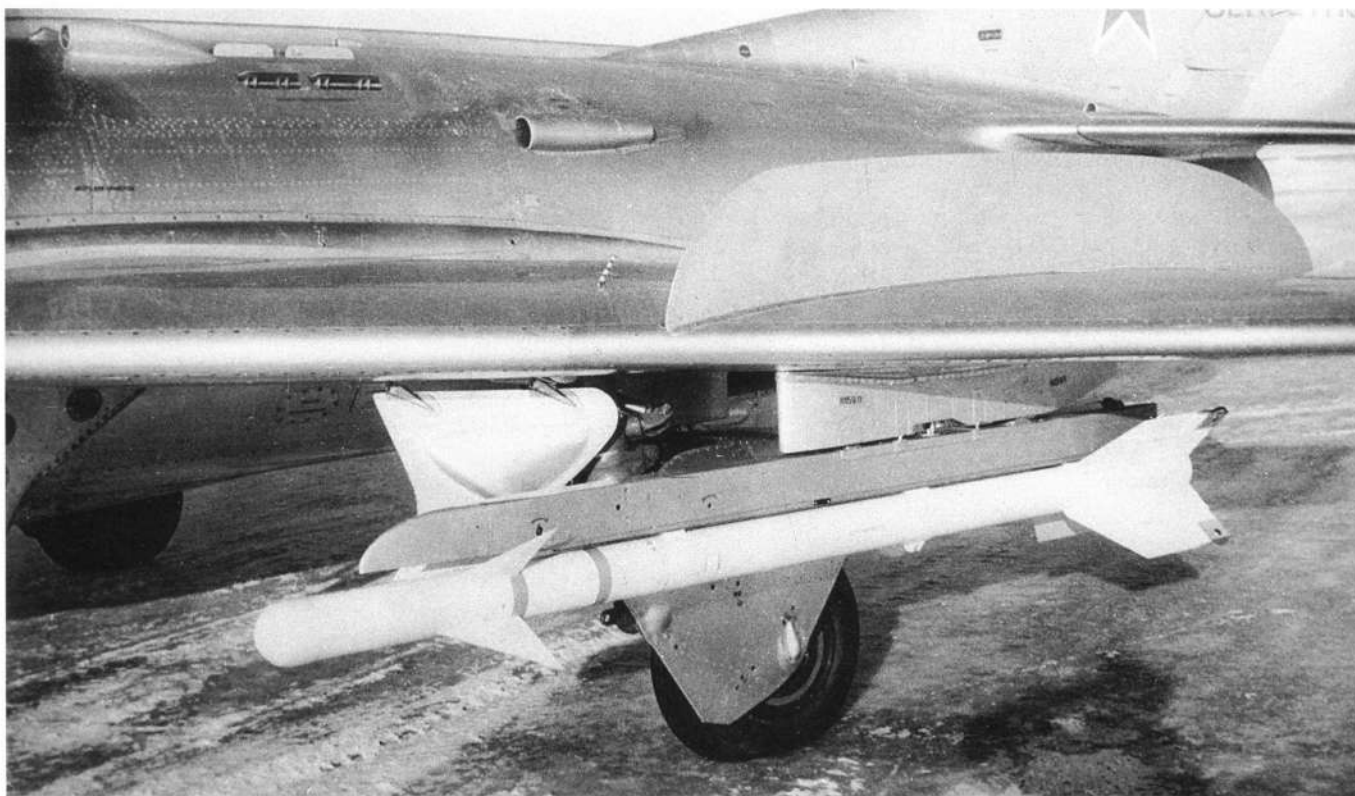
Ракета К-13 из опытной серии под крылом истребителя МиГ-19, 1959 год
