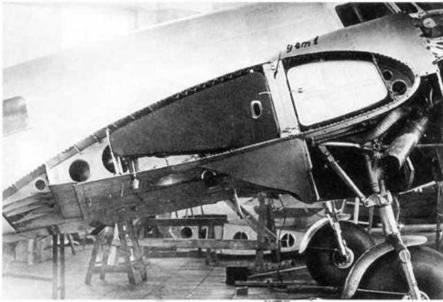
Разобранная «Электра» в цехе завода № 156 в Москве (предоставлено Г.Слуцким)
