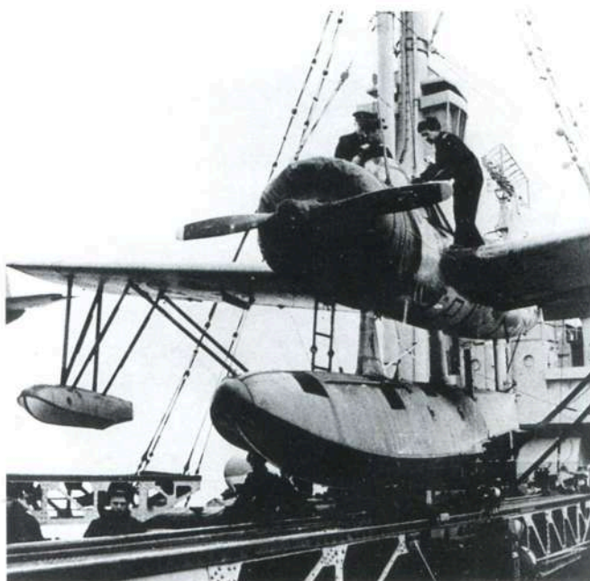
«Кингфишер» на катапульте крейсера «Мурманск» во время его приемки на Северном флоте (предоставлено В.Рыбиным)
