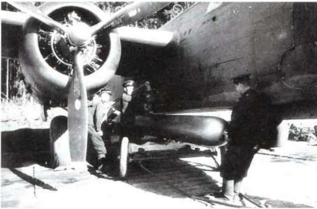
Подвеска торпеды 45-36-АН на правый торпедный мост «Бостона», самолет Героя Советского Союза А.М.Гагинева
