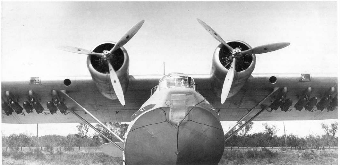
Опытный образец военного ГСТ с вооружением на испытаниях в НИИ морской авиации. Хорошо видна громоздкая цилиндрическая носовая турель, совершенно не похожая на американскую коническую
