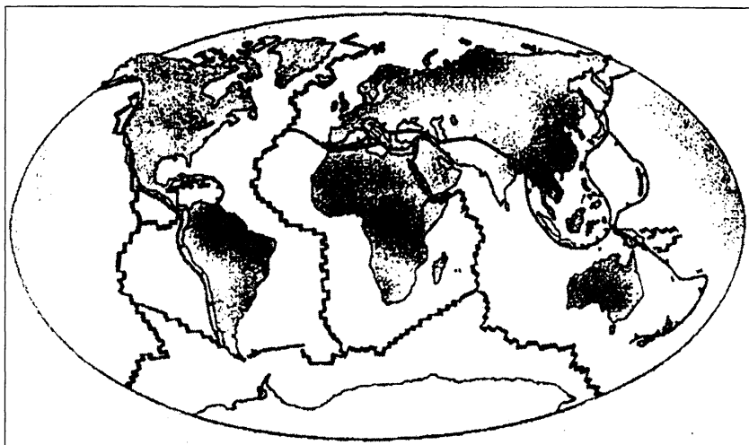
Рис. 4. Карта трещин и разломов земной коры
