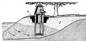
Рис. 3. Инфильтрационный колодезь: 1 — песок; 2 — гравий; 3 — водоупорный слой; 4 — глиняный замок.
