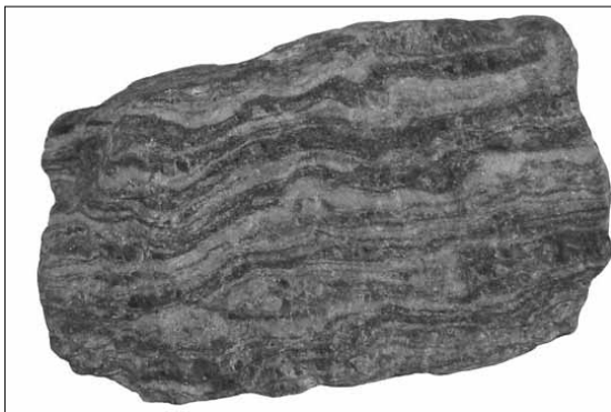
Гнейс, метаморфическая порода
