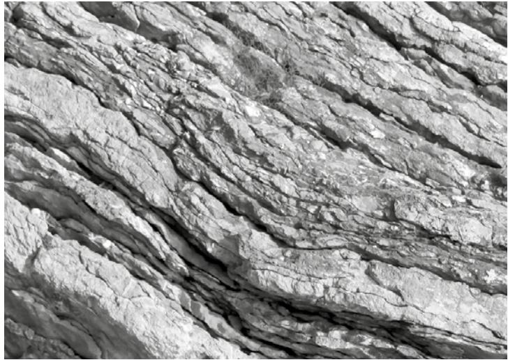
Осадочные породы залегают стратами
