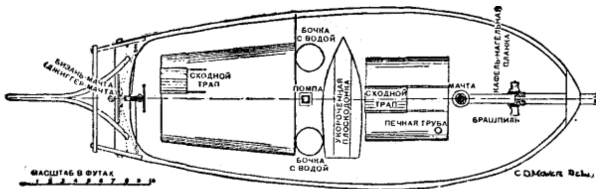
План палубы "Спрея"
