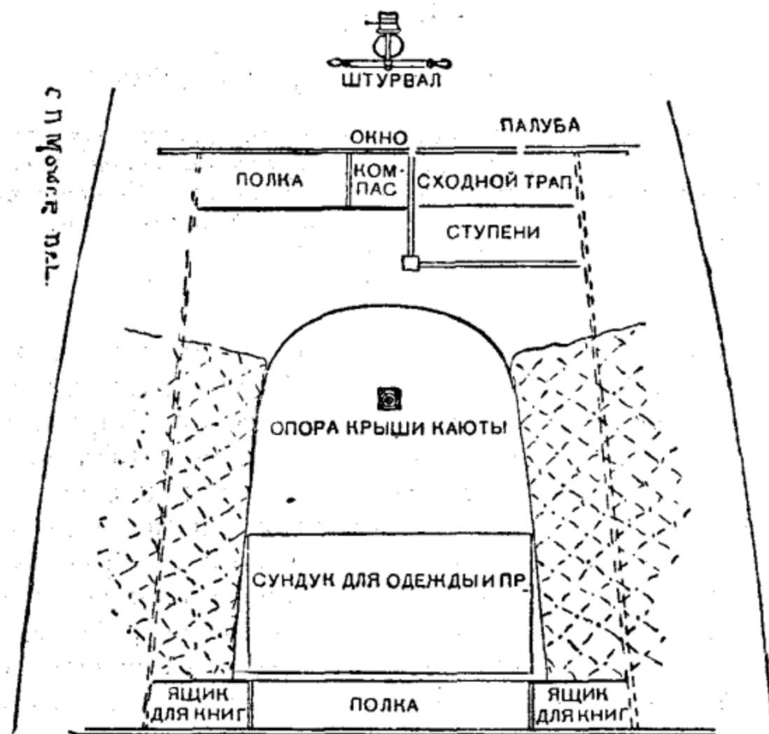
План каюты на „Спрее“
