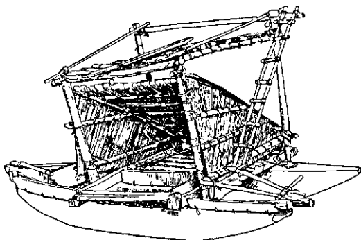
Судно для плаванія въ открытомъ морѣ, бывшее нѣкогда въ употребленіи на островахъ Самоа.
