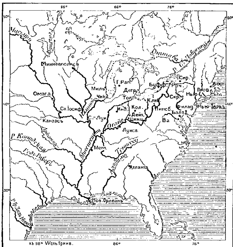
№ 539. Судходныя рѣки Сѣверной Америки.
