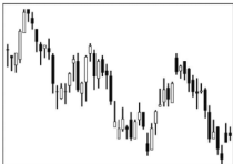
Рис. 12.14. Свечной график
