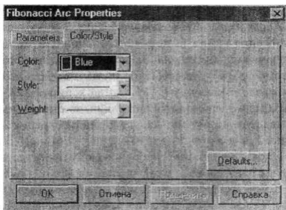
Рис. 29. Страница цвета/стиля
