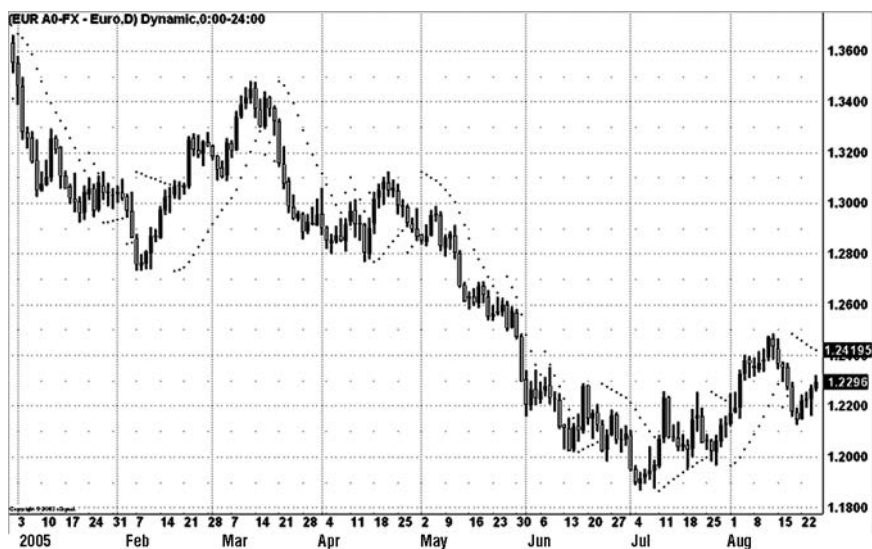
РИС. 7.3. Параболический SAR
