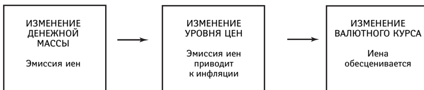
РИС. 3.5. Монетарная модель
