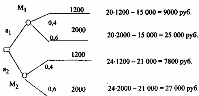
Рис. 2.2. Дерево решений
