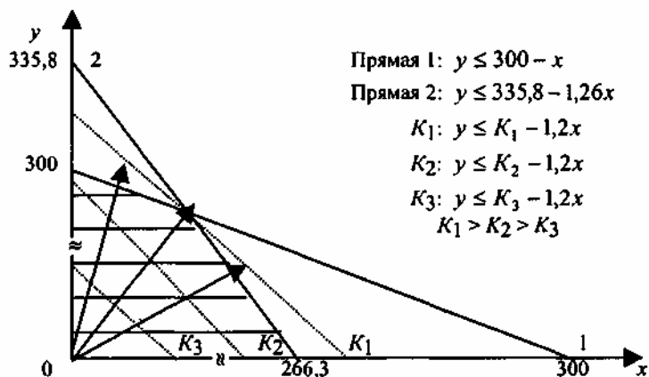
Рис. 2.3. Поиск решения задачи линейного программирования
