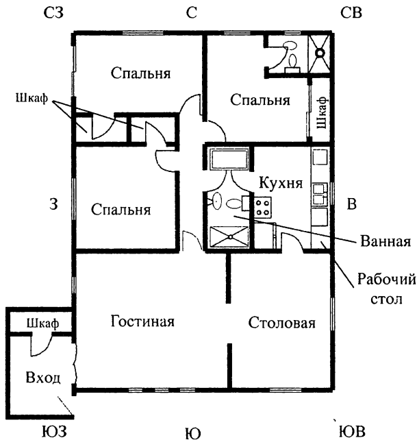
Рис. 3-15. Дом с расширенным юго-западным сектором
