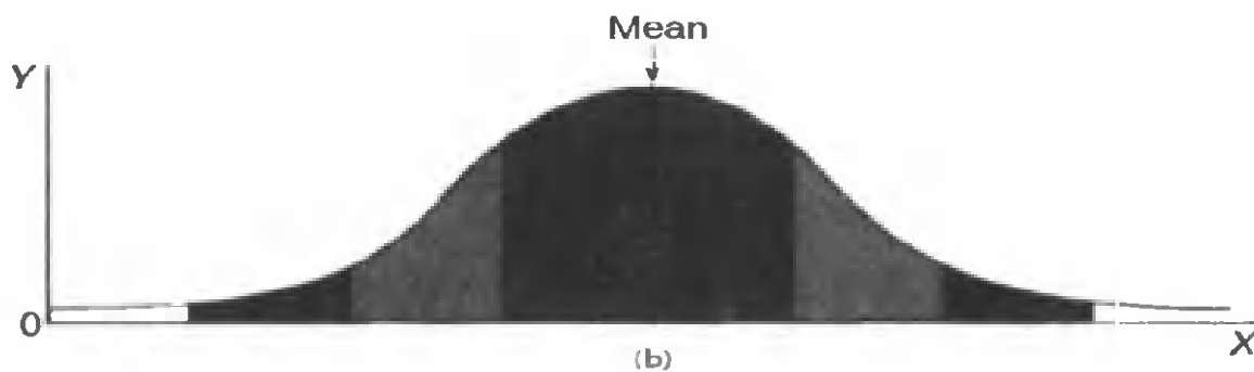
Рис. 3.6. Примеры малого (a) и большого (b) стандартного отклонения.
