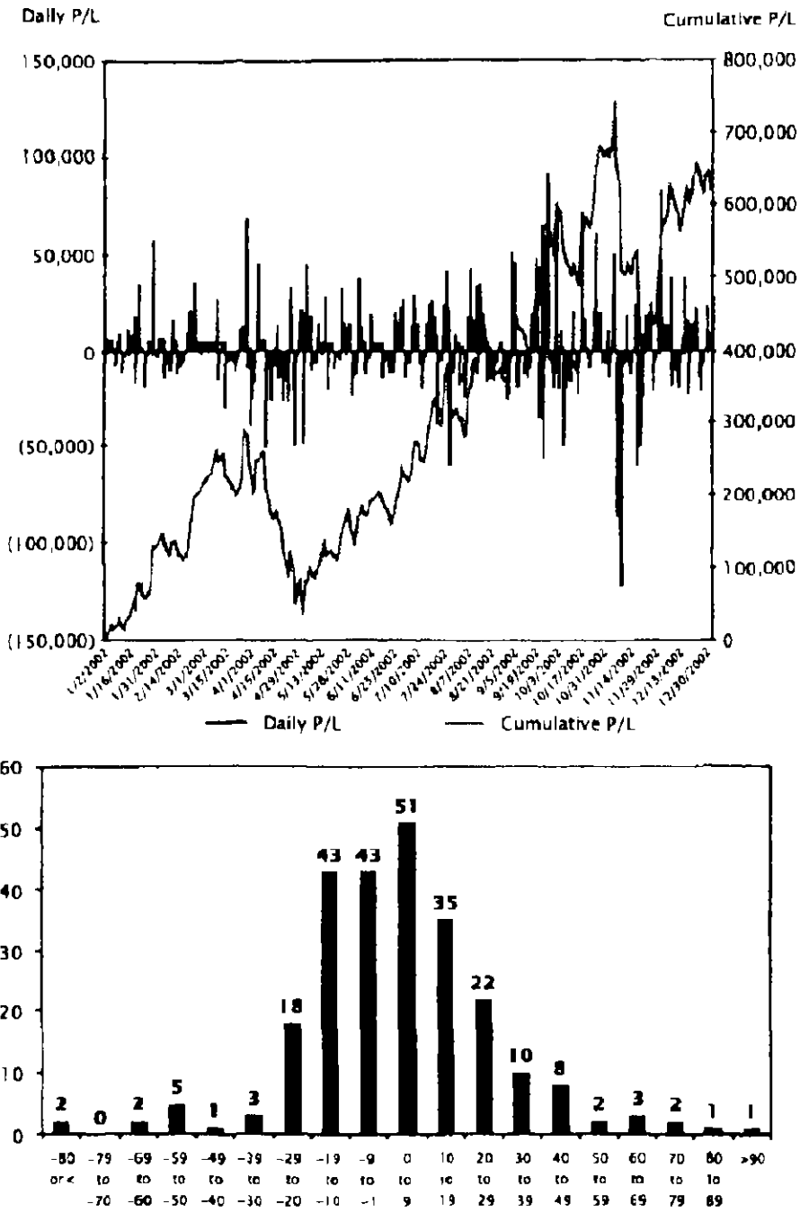
Рис. 3.7. Пример сводки статистических данных.
