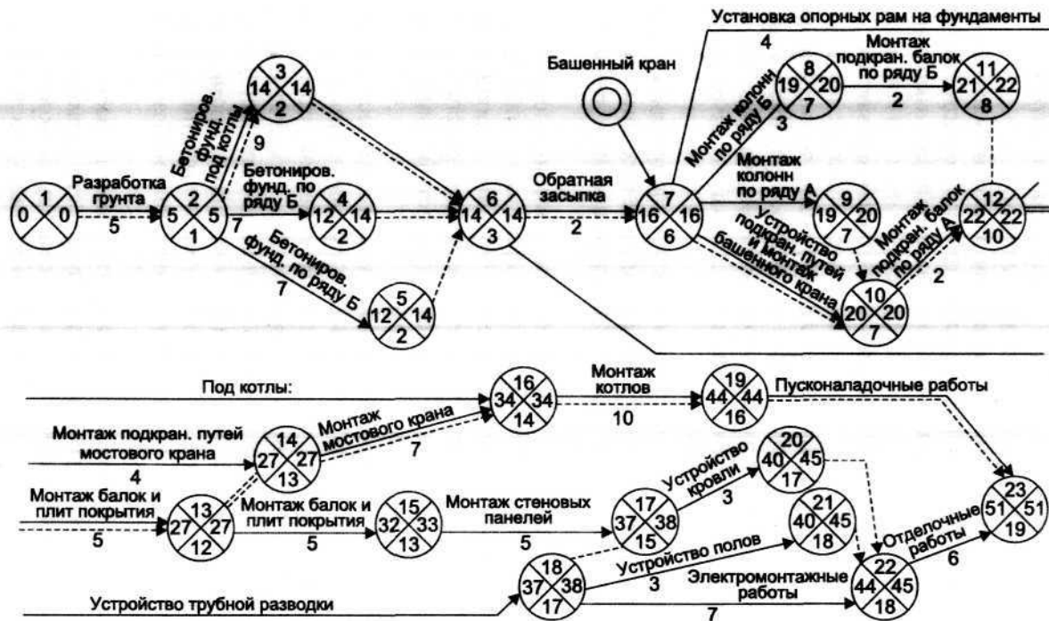
Рис. 6.1. Сетевой график строительства котельной. Обозначения: каждый круг считается одной из вершин графика; цифра в верхнем секторе каждой вершины означает ее порядковый номер; из номеров двух соседних вершин складывается шифр работы; цифра в нижнем секторе каждой вершины является порядковым номером предшествующей вершины, а линия, соединяющая эти две вершины, означает определенную работу. Внизу под линией записана плановая продолжительность данной работы; цифра в левом секторе каждой вершины означает общую продолжительность всех предшествующих работ, цифра в правом секторе отличается от цифры в левом на величину резерва (запаса времени). Таким образом, для вершин, лежащих на критическом пути, цифры в левом и правом секторах вершины совпадают, поскольку запас времени равен 0.
