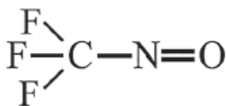
Трифторнитрозометан (XIX)
