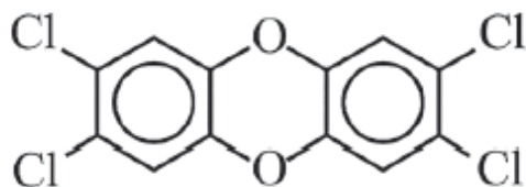
2,3,7,8-Тетрахлордibenзо-п-диоксин (XXIX)
