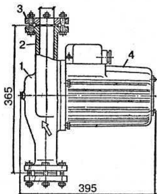
Рис. 6. Центробежный циркуляционный насос типа ЦВЦ:
