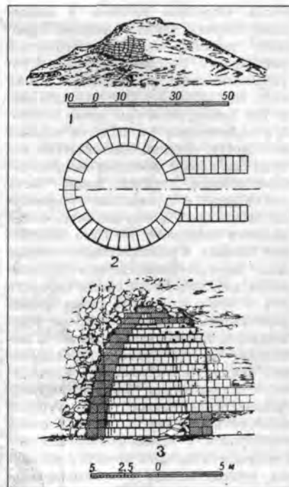
Золотой курган близ Керчи: 1 — общий вид; 2 — план склепа; 3 — продольный разрез склепа
