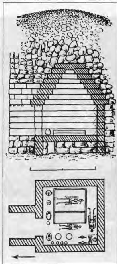
Погребение в кургане Куль-Оба (план и разрез)
