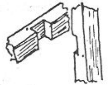
Замок прилонный
