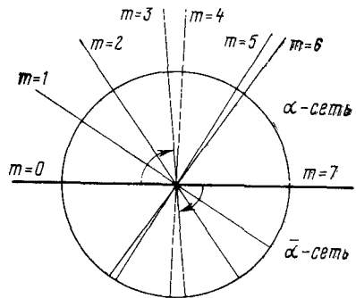
Рис. 2.12. Диаграмма распределений мощностей в цепи из семи ветвей, структура различных соединений которых представлена на рис. 2.3.
