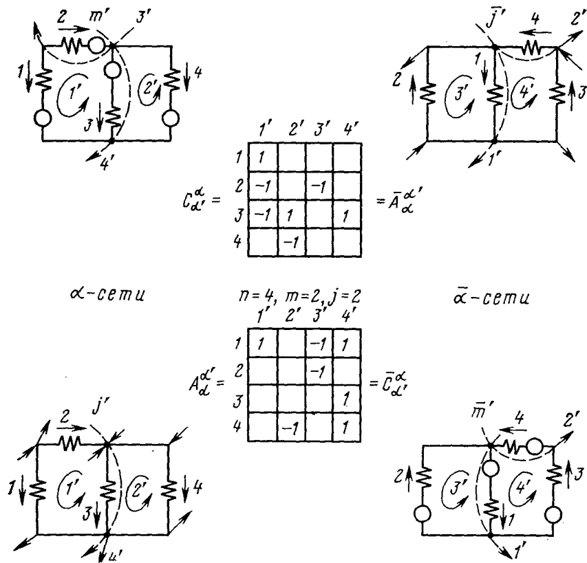
Рис. 2.11. Пример цепей из четырех ветвей с двойственными в смысле матриц преобразования структурами, а также соответствующие им матрицы преобразования
