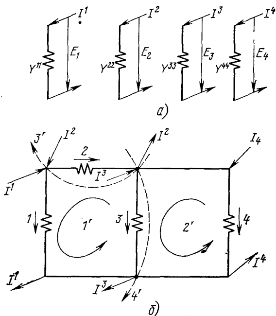
Рис. 2.5. Величины на ветвях электрической цепи при возбуждении источниками тока: а — простейшая цепь из четырех отдельных ветвей, возбуждаемых источниками тока I^\alpha б — те же ветви, соединенные в структуру, выбор замкнутых и разомкнутых путей в этой структуре, величины на отдельных ветвях
