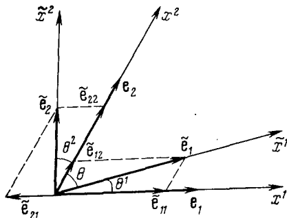
Рис. 1.5. Преобразование векторов базиса при переходе от системы координат (x^1, x^2) к системе координат (\bar{x}^1, \bar{x}^2)
