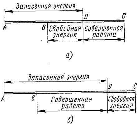
Рис. 1.10. Энергия в конденсаторе (или в электромагните): а — постоянный заряд (или поток); б — постоянная э. д. с. (или м. д. с.)
