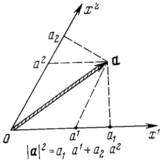
Рис. 1.9. Выражение квадрата длины вектора \mathbf{a} через ковариантные и контравариантные компоненты
