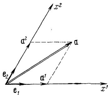
Рис. 1.4. Разложение вектора a по векторам компонентам базиса в системе координат (x^1, x^2) двумерного аффинного пространства
