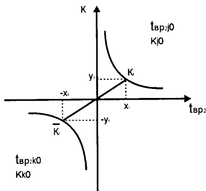
Рис. 28 Область положительных и отрицательных значений функции K=1/t_{вр2}
