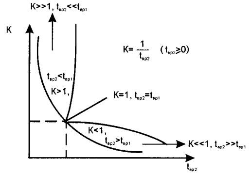
Рис. 7 График зависимости K=1/t_{\text{вр}}^2
