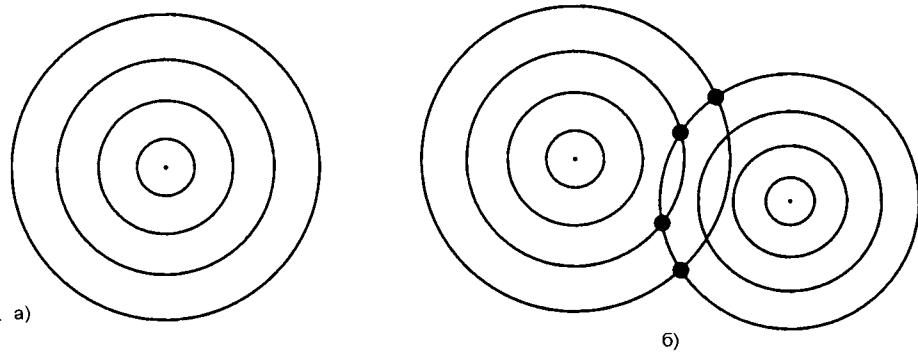
Рис. 18 Поле точечных акустических источников а) для одиночного источника б) для двух точечных источников
