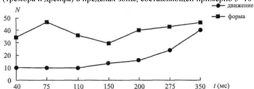
График 6. Результаты порождения формы и движения движущегося объекта, показанные испытуемым 1 (суммарно по 7-й и 8-й сериям)
