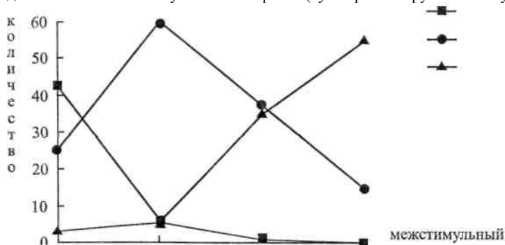
График 3. Порождение движения и стабильности в стробоскопических условиях восприятия в зависимости от длительности межстимульного интервала (суммарно по группе испытуемых и по всем тест-объектам)
