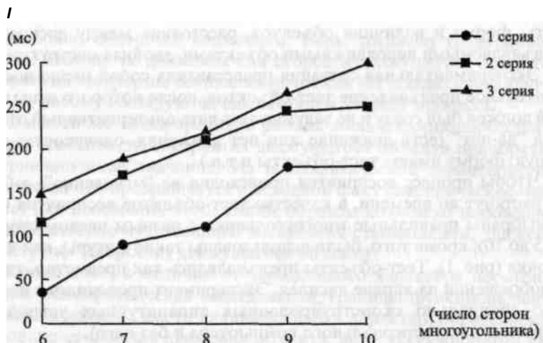
График 1. Критическое время формопорождения (КВФ) объектов (6, 7, 8, 9 и 10-многоугольников) при их неподвижности - 1 серия, при их фронтальном движении со скоростью 7 угл.град./с. - 2 серия, и 14 угл.град./с. - 3 серия (усредненные данные)
