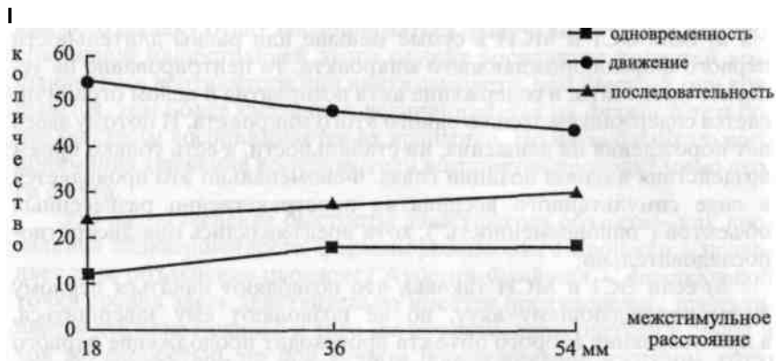
График 4. Порождение движения и стабильности в стробоскопических условиях восприятия в зависимости от пространственной разнесенности тест-объектов (суммарно по группе испытуемых и по всем тест-объектам)
