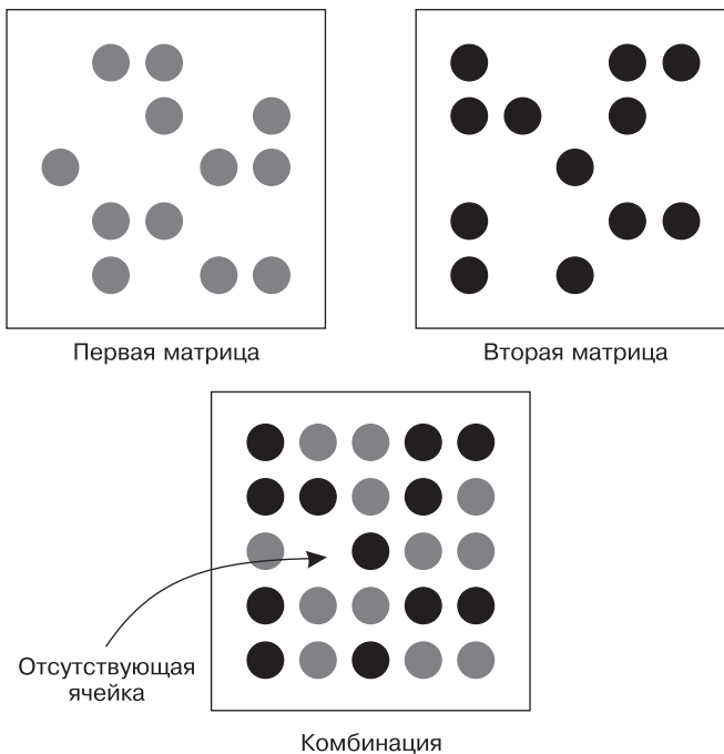
Рис. 32. Псевдослучайные матрицы
