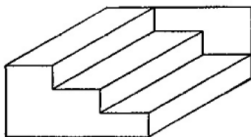
Рис. 2. Лестница Шредера
