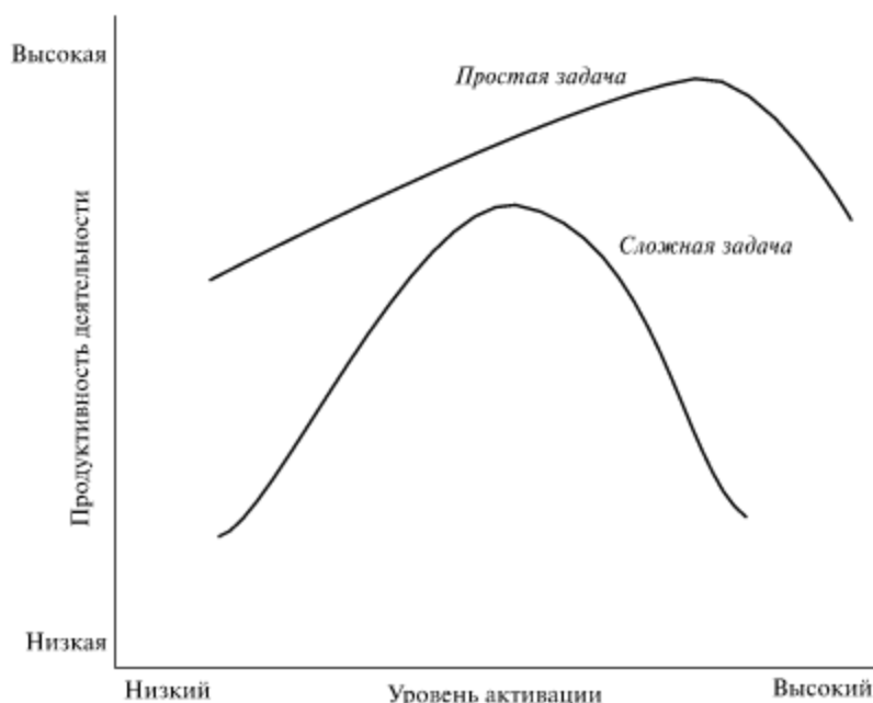
Рис. 2. Закон Йеркса—Додсона 3
