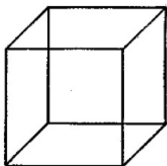
Рис. 1. Куб Неккера
