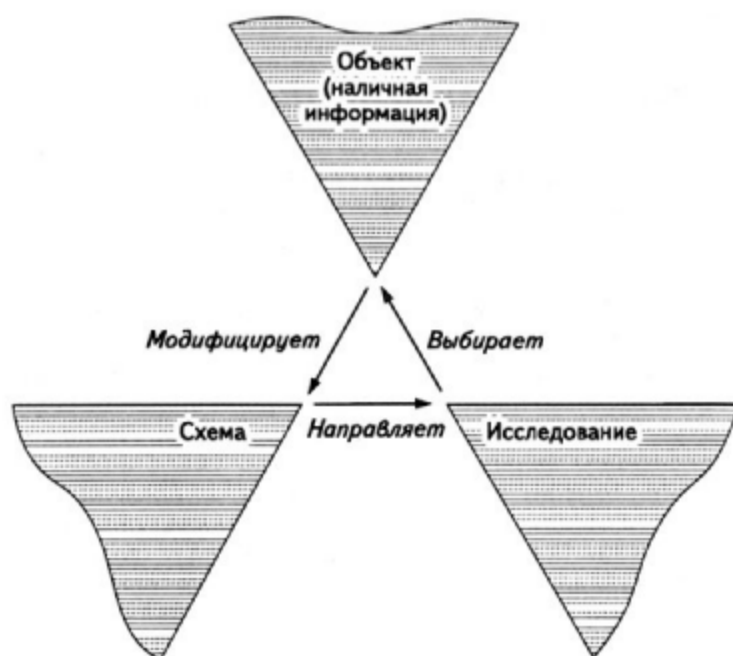
Рис. 1. Перцептивный цикл 7
