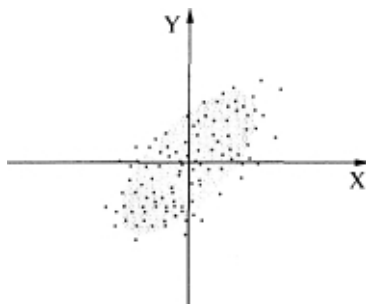
Рис 12.1. Диаграмма рассеивания.
