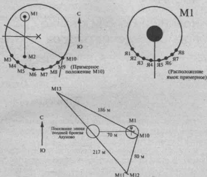
Рис. 25. Схема расположения менгиров в Ахуновском святилище (по данным экспедиции Ф.Н. Петрова)
