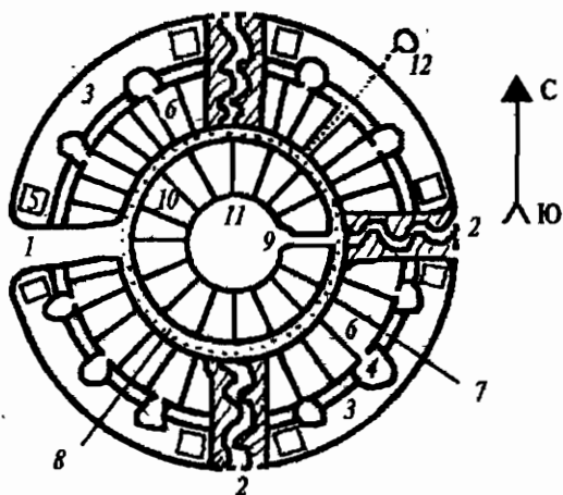
Рис. 18. Схема внутренней оборонительной системы:
