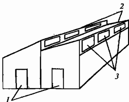
Рис. 20. Схема освещения аркаимского жилища: 1 — входные двери; 2 — наклонные крыши; 3 — проемы для окон
