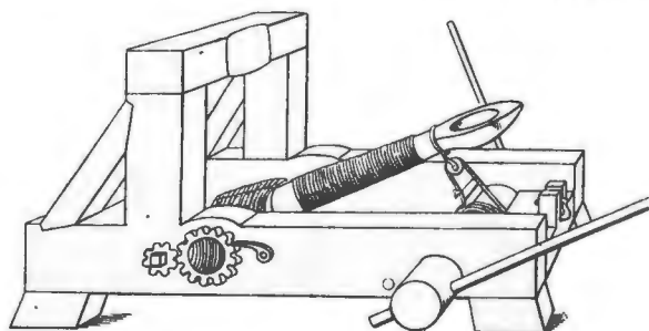
202. Камнеметъ или баллиста.
