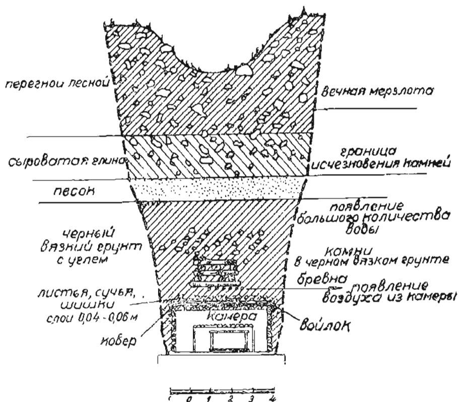
Рис. 4. Разрез по вертикали кургана № 6 (Ноин-ула).
