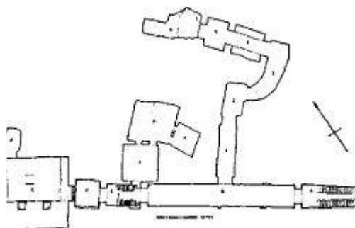
План царской гробницы в эль-Амарне.
