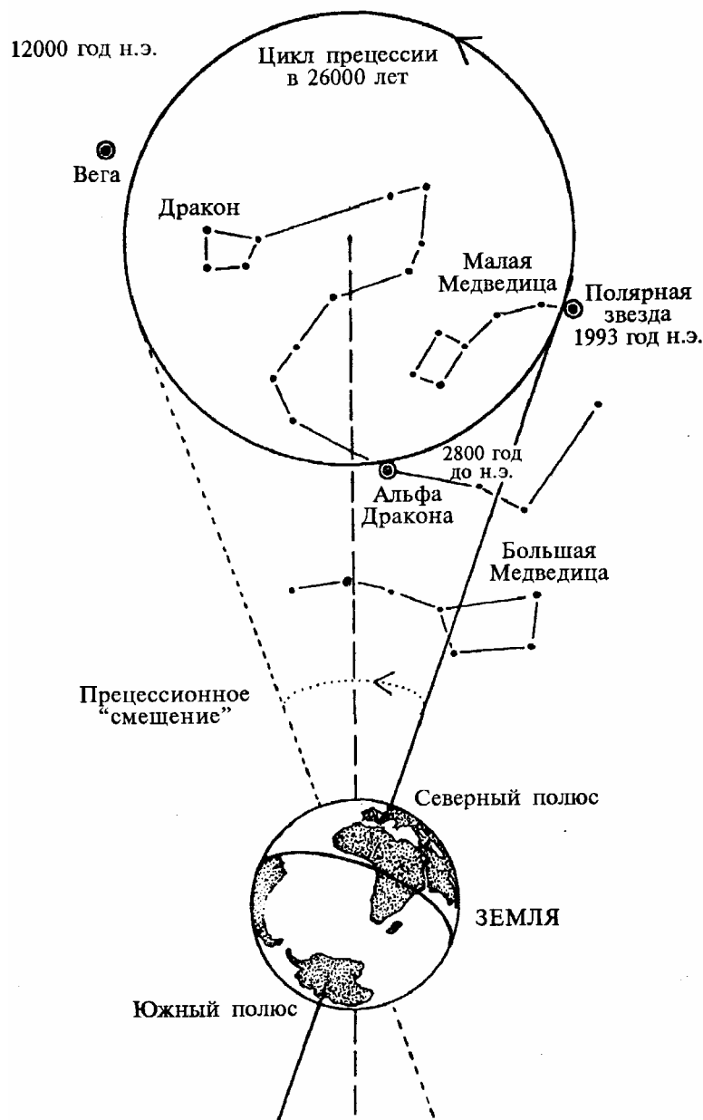
24. Прецессия
