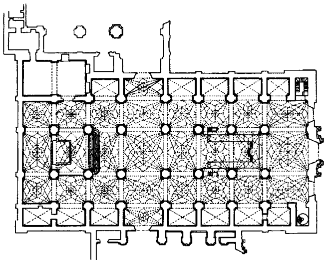
План собора Куско
