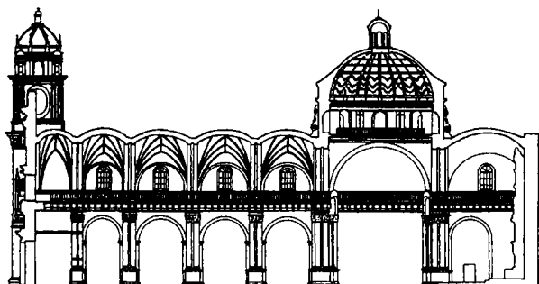
Церковь иезуитов в Куско, продольный разрез
