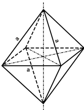
Рис. 3.18. Кристаллическая структура алмаза
