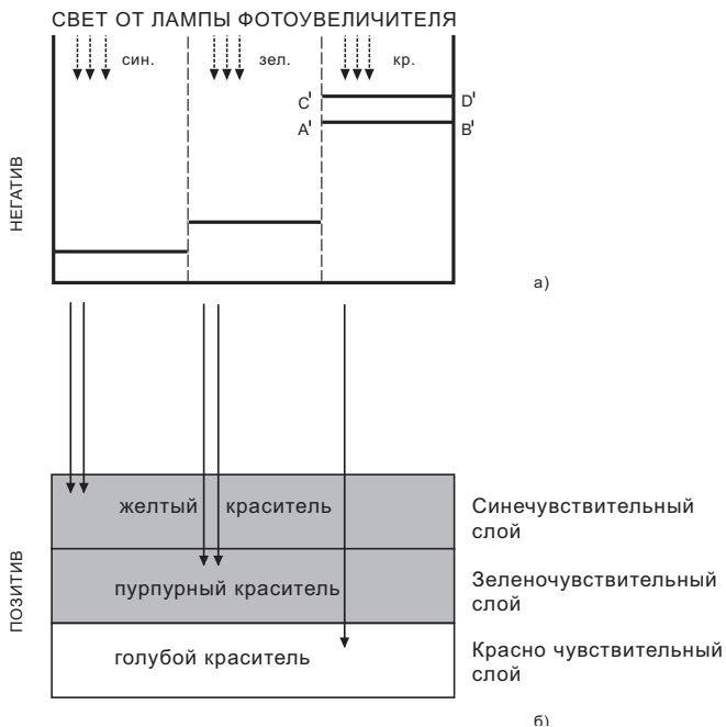
Рис 12. Схематическое изображение процесса печати голубого негативного красителя (а) на цветную фотобумагу (б)
