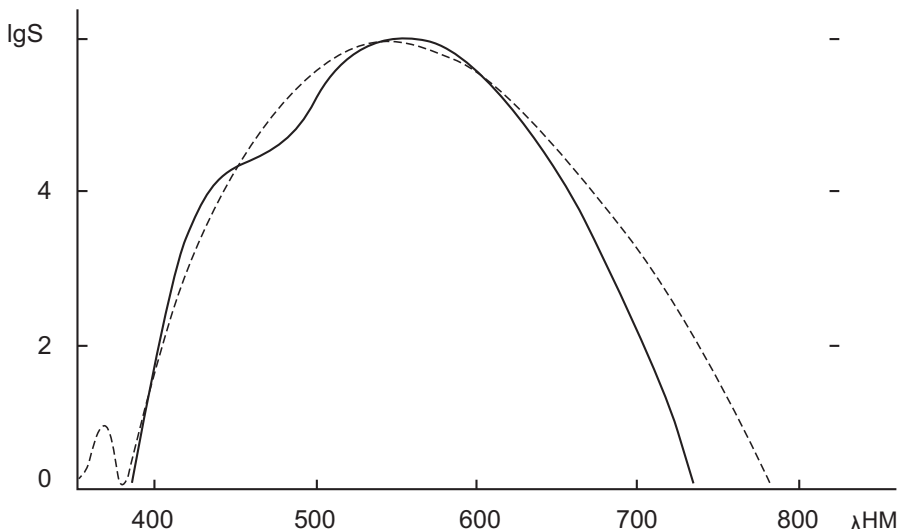
Рис 5. Спектральный ответ денситометра со светофильтром Кодак Рэттен W-106 (—) и колориметрическая функция смешения цветов \Upsilon_{\lambda} в системе МКО 1931 г. для источника света с цветовой температурой 3200 К (---) 1 .
