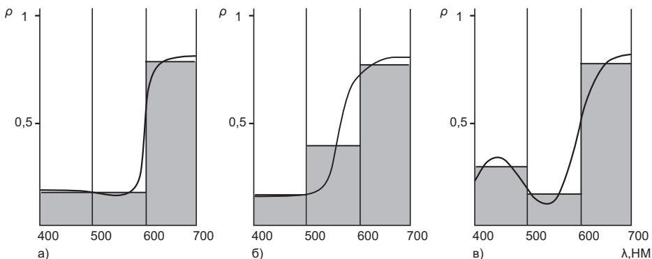
Рис 21. Спектральные кривые отражения красного (а), оранжевого (б) и пурпурного (в) полей в трехзональной диаграмме
