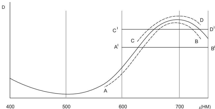
Рис 10. Спектральная характеристика поглощения голубого красителя фотоплёнок
