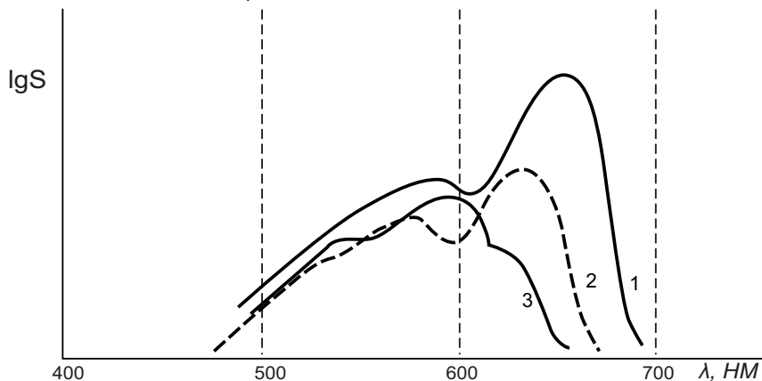
Рис 50. Кривые фотоактивных потоков спектральных сенсibilизаторов 3554 (1), 6089 (2) и 4012 (3)
