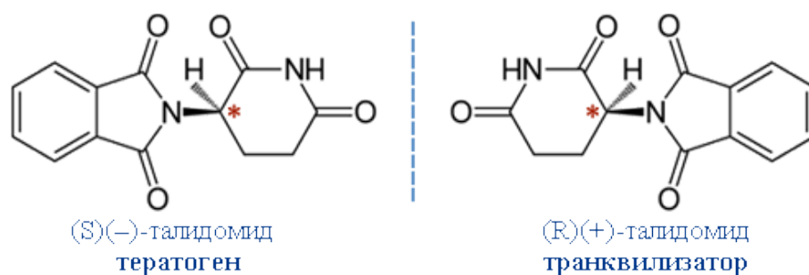
Рис. 5.4. Энантимеры талидомида
