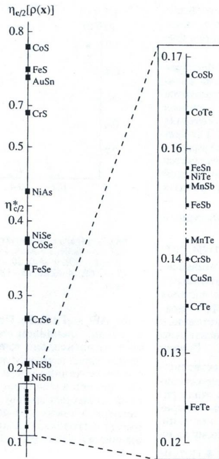
Рис. 2. \eta -диаграмма структурного типа арсенида никеля – пирротина
