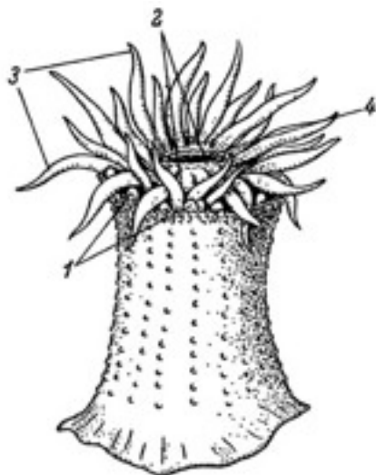
Строение актинии (по Наумов, 1976): 1 - акрохаги, 2 - оральный диск, 3 - щупальца, 4 - ротное отверстие
