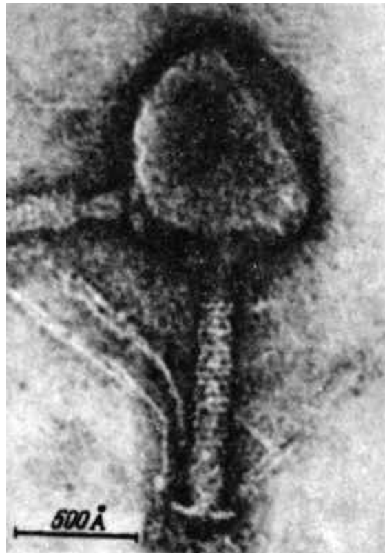
Рис. 8 Электронная микрофотография одного из сложных бактериальных вирусов – фага T2. Хорошо видны молекулы белка, слагающие хвост и голову, а также хвостовые нити (слева). Размеры здесь также в ангстремах.
