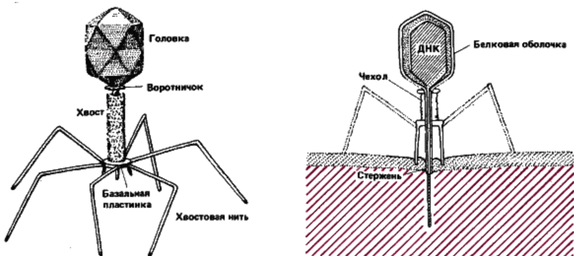
Рис. 9. Подробная схема Т-четного фага; справа показано, как он заражает бактерию.
