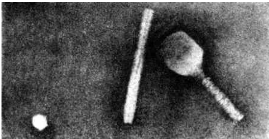
Рис. 6. Относительные размеры некоторых вирусов (электронная микрофотография с
