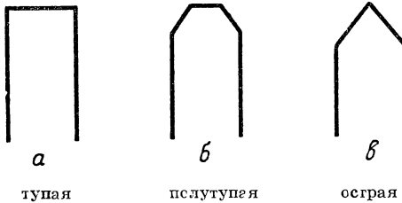
Рис. 14. Профиль линеек.
