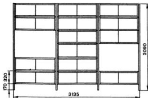
Рис. 10. Трехсекционный книжный стеллаж
