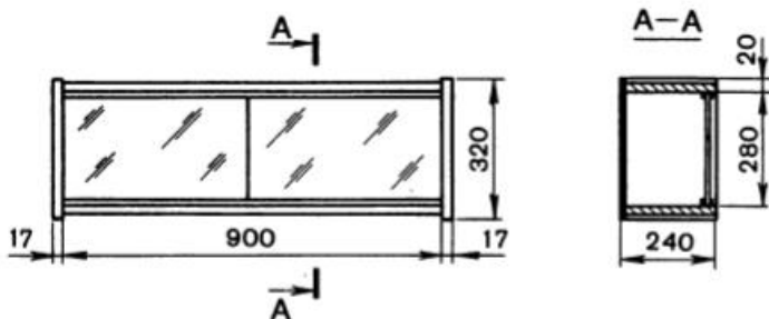
Рис. 9. Одноярусная книжная полка
