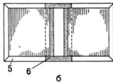
Рис. 3. Переплетные крышки: а) цельнотканевая: 1) картонные сторонки, 2) отстав, 3) покровный материал 4) расстав; б) составная, 5) бумажная или другая ткань, 6) корешковый материал
