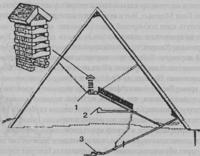
Вертикальный разрез пирамиды Хеопса
