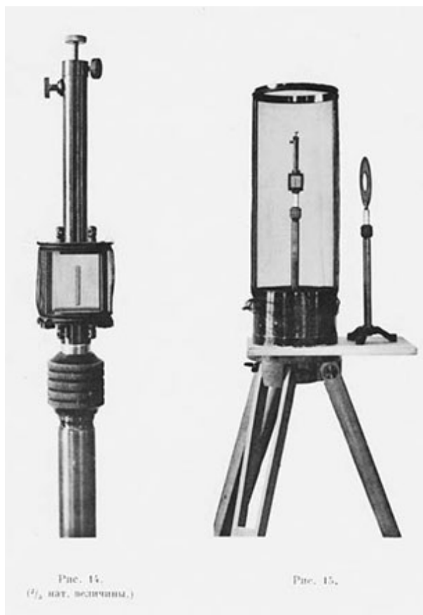
Портативный фонометр Лебедева - Зёрнова (общий вид).
