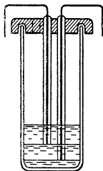
Сосуд Аррениуса для определения электропроводности растворов
