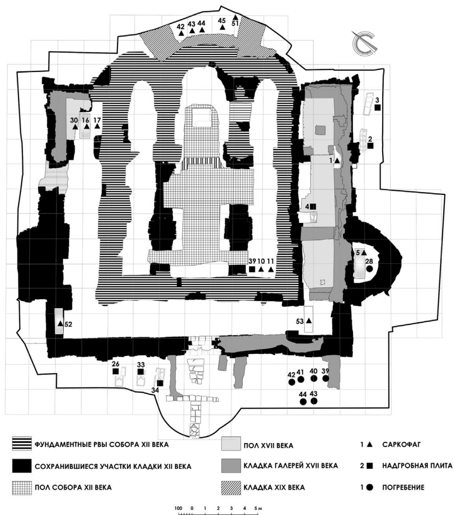
Рис. 1. Обобщенный план работ 1997-2000 гг. с указанием основных погребений
