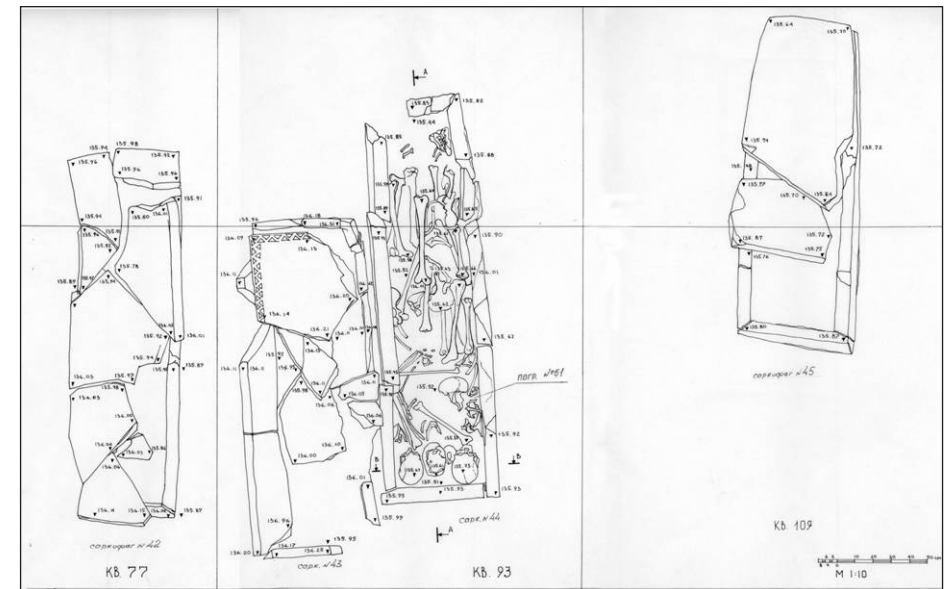
Рис. 18. Группа саркофагов к востоку от апсиды, часть обмерного плана
