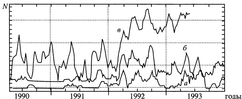
Число авиакатастроф (а), пожаров на складах сырья и промышленных предприятий (б) в России в сопоставлении с числами Вольфа (в)
