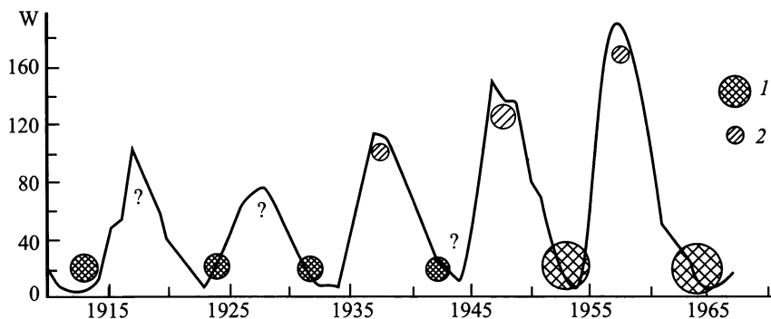
Время развития эпизоотических волн в природных очагах чумы в зависимости от хода изменений солнечной активности: 1 – 10-11-летние, 2 – 4-5-летние эпизоотические волны
