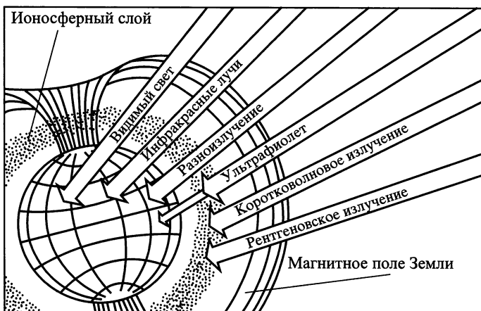
Физические факторы космического воздействия на Землю
