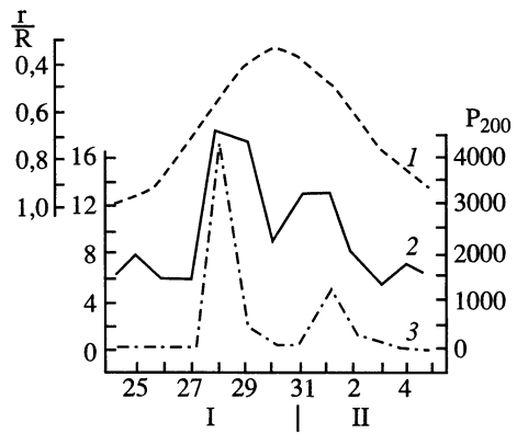
Солнечная активность (1) и общая онкологическая заболеваемость в Туркменской ССР (2)
