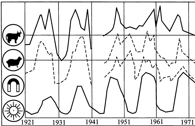
Изменения поголовья мелкого рогатого скота и коров в связи с колебаниями магнитной и солнечной активности (по Д.И. Маликову)
