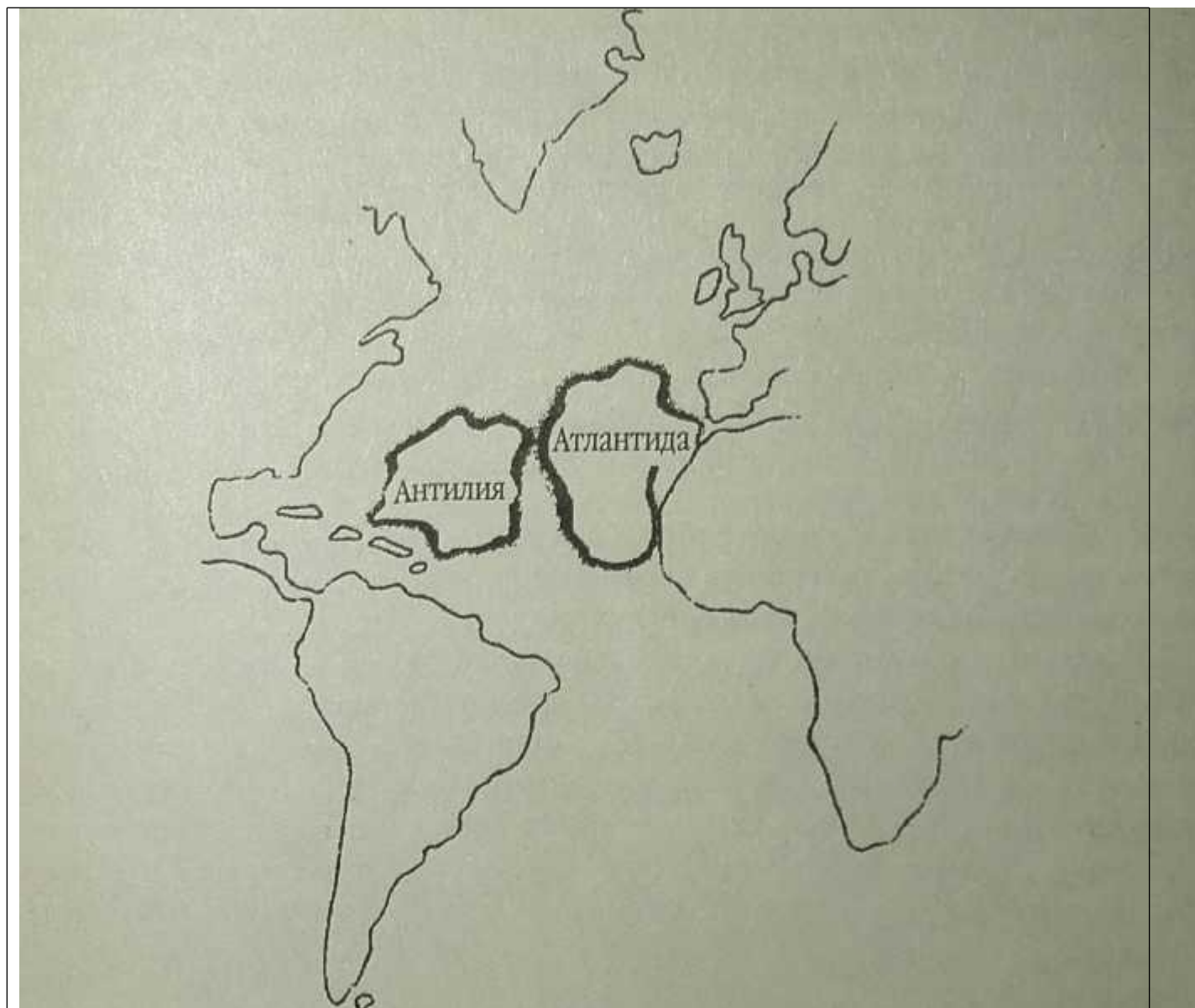
Рисунок 6. Положение двух островов согласно Льюису Спенсу.
