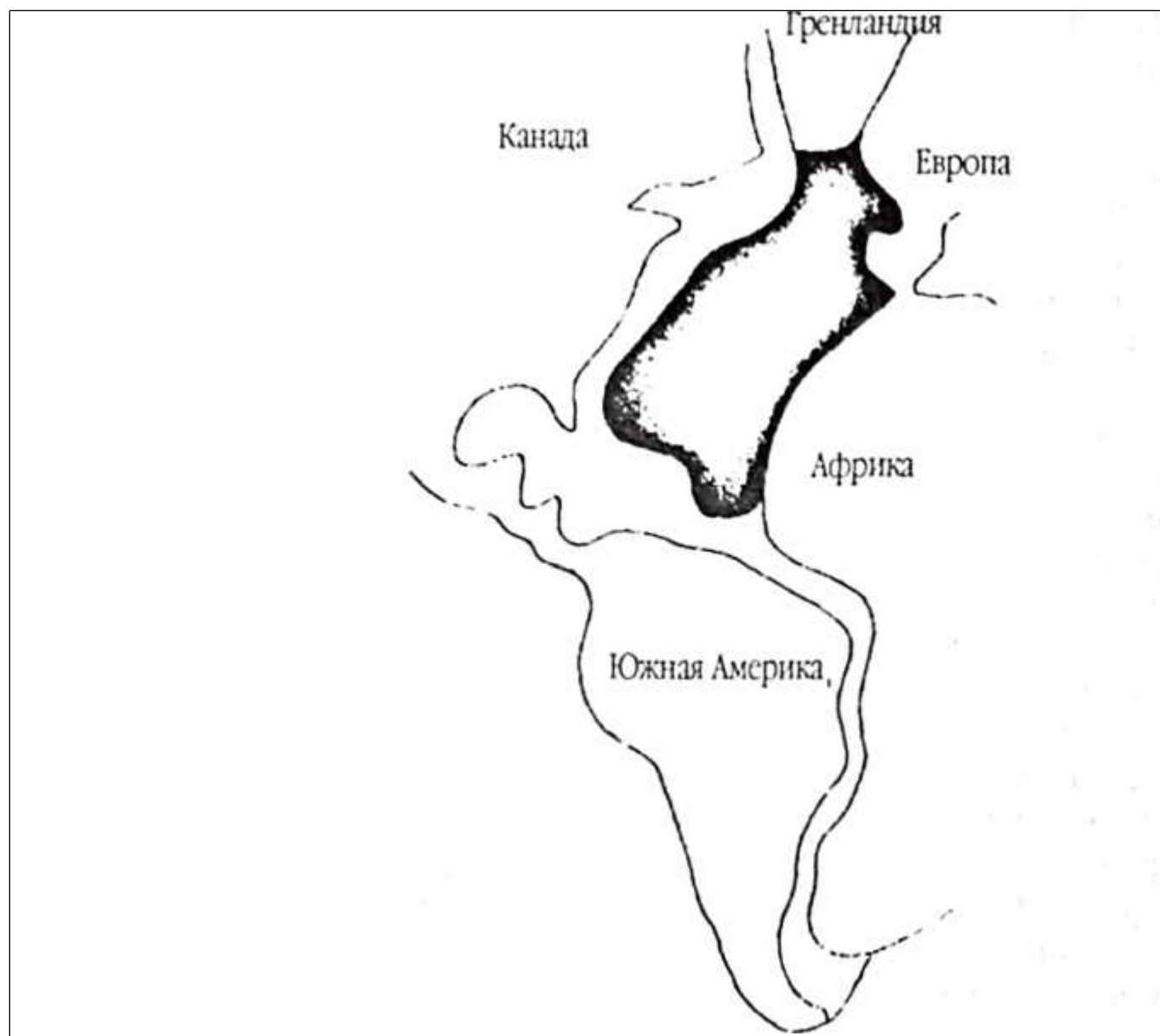
Рисунок 2. Из рисунка видно, что материковые шельфы не соответствуют друг другу в области Северной Атлантики, хотя ближе к югу они хорошо описываются теорией Вегенера.
