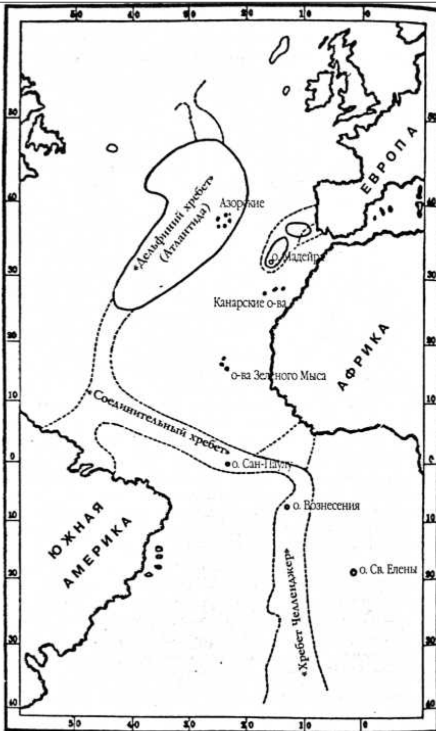
Рисунок 11а. Карта Атлантиды с ее островами и соединительными хребтами, полученная в результате глубоководного зондирования.
